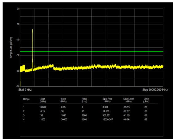
n38 SCS=30kHz CP_QPSK BW=40MHz Channel=520000 RB=106@0
