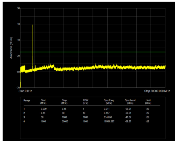
n38 SCS=30kHz DFT_QPSK BW=20MHz Channel=516000 RB=50@0
