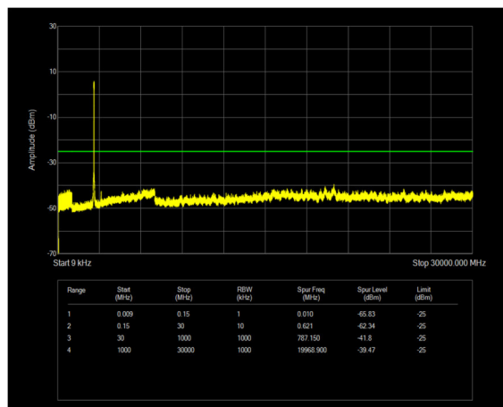
n38 SCS=30kHz DFT_QPSK BW=40MHz Channel=520000 RB=100@0
