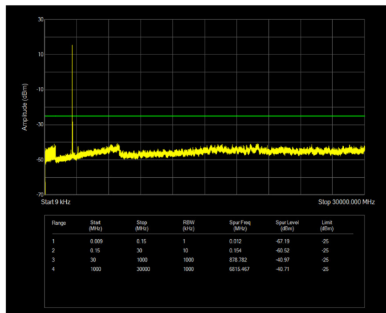
n38 SCS=30kHz CP_QPSK BW=40MHz Channel=520000 RB=1@0
