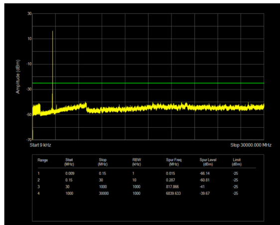
n38 SCS=30kHz CP_QPSK BW=40MHz Channel=518000 RB=1@105
