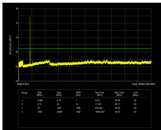
n38 SCS=30kHz DFT_QPSK BW=40MHz Channel=519000 RB=1@0
