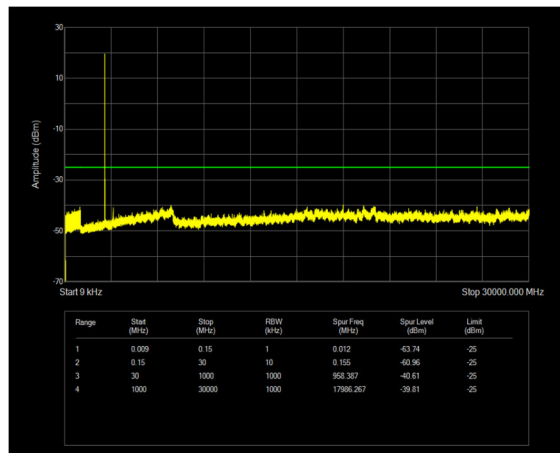
n38 SCS=30kHz DFT_QPSK BW=20MHz Channel=516000 RB=1@0
