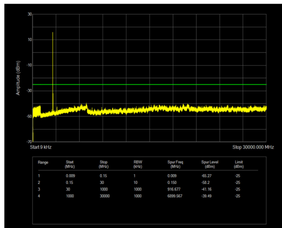
n38 SCS=30kHz CP_QPSK BW=40MHz Channel=518000 RB=1@0
