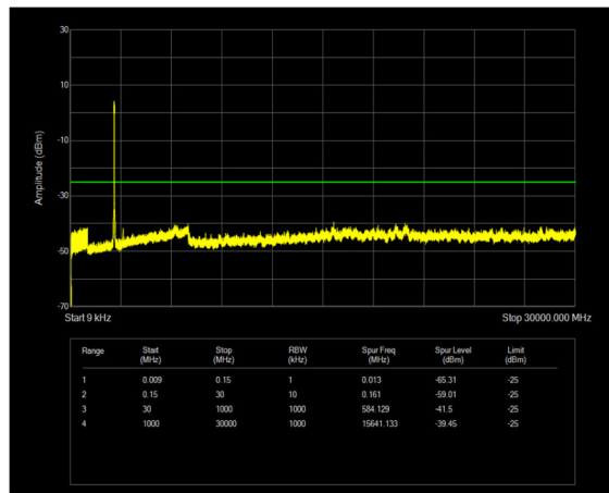
n38 SCS=30kHz CP_QPSK BW=40MHz Channel=519000 RB=106@0
