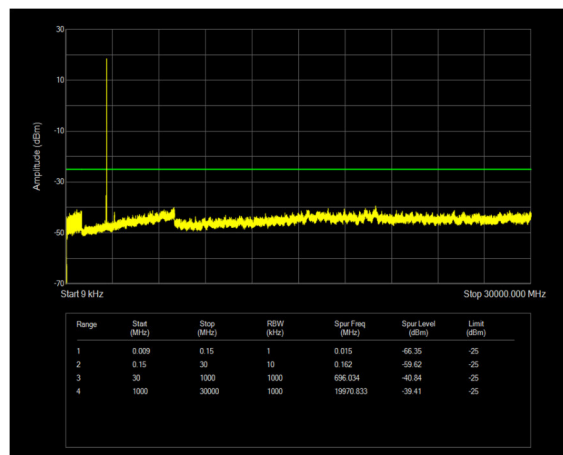
n38 SCS=30kHz DFT_QPSK BW=40MHz Channel=519000 RB=1@105
