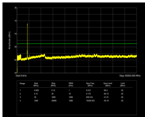
n38 SCS=30kHz DFT_QPSK BW=40MHz Channel=519000 RB=100@0
