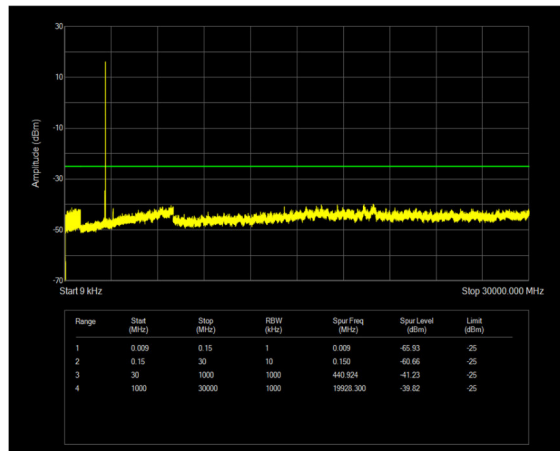
n38 SCS=30kHz CP_QPSK BW=40MHz Channel=519000 RB=1@105
