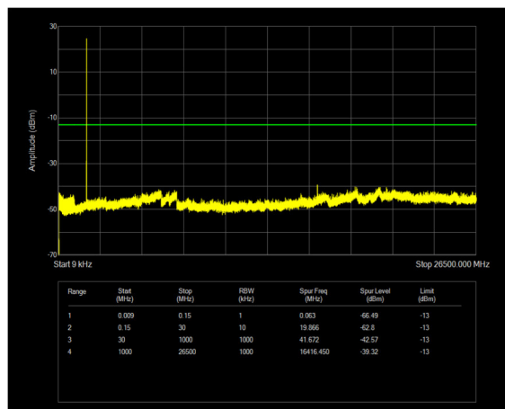
n66 SCS=15kHz DFT_QPSK BW=20MHz Channel=354000 RB=1@105
