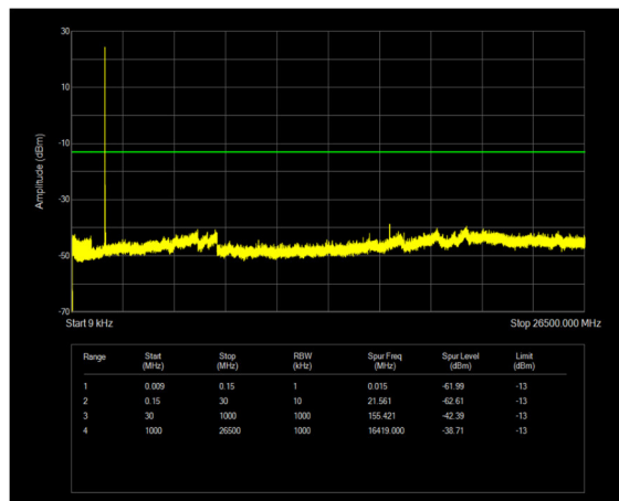
n66 SCS=15kHz DFT_QPSK BW=20MHz Channel=344000 RB=1@0
