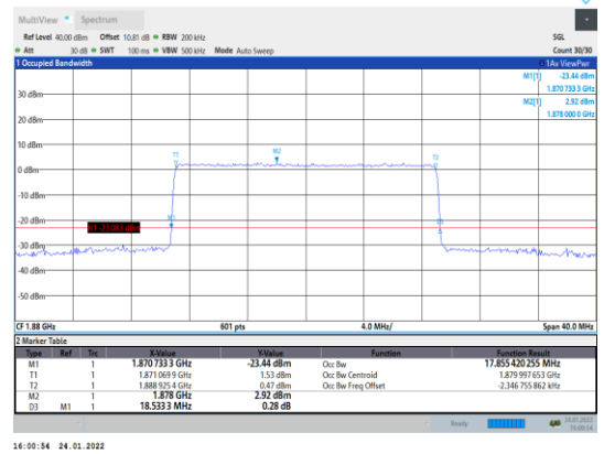
Band2-20MHz-16QAM-18900-100RB#0
