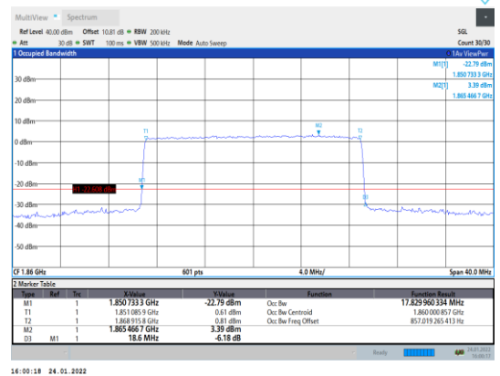
Band2-20MHz-16QAM-18700-100RB#0
