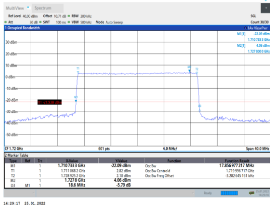
Band4-20MHz-QPSK-20050-100RB#0
