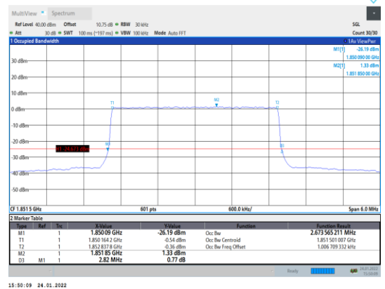
Band2-3MHz-16QAM-18615-15RB#0
