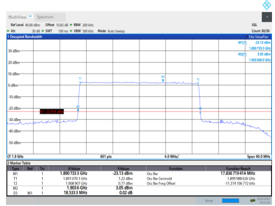
Band2-20MHz-16QAM-19100-100RB#0
