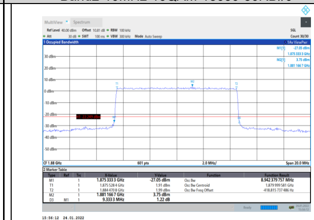
Band2-10MHz-16QAM-18900-50RB#0
