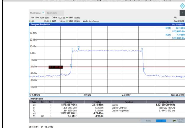
Band2-10MHz-QPSK-18900-50RB#0
