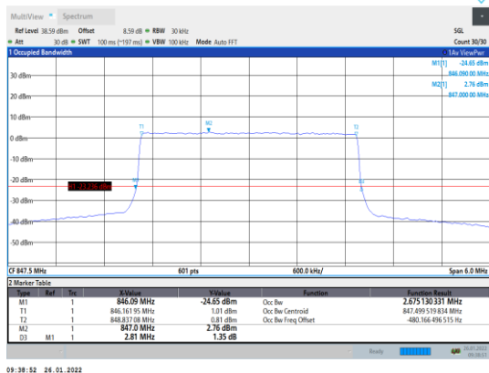
Band5-3MHz-QPSK-20635-15RB#0
