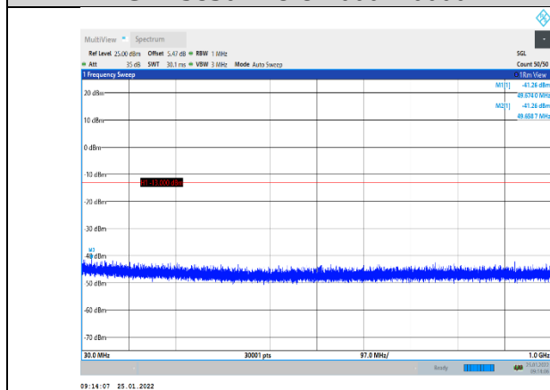
EGPRS850-190-8-30~1000MHz
