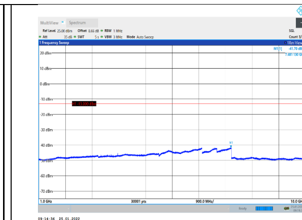
EGPRS850-190-8-1000~10000MHz
