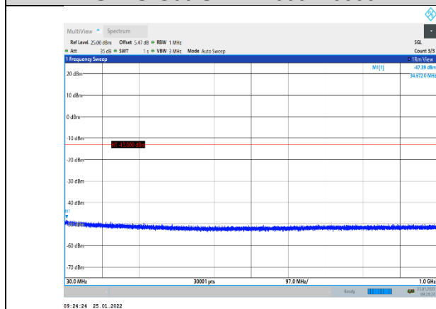
EGPRS1900-661-2-30~1000MHz
