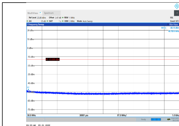
EGPRS1900-512-2-30~1000MHz
