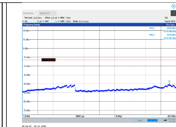
EGPRS1900-661-2-1000~20000MHz
