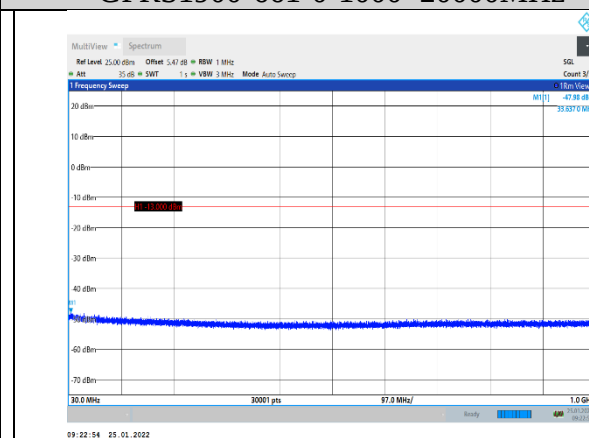
GPRS1900-810-0-30~1000MHz
