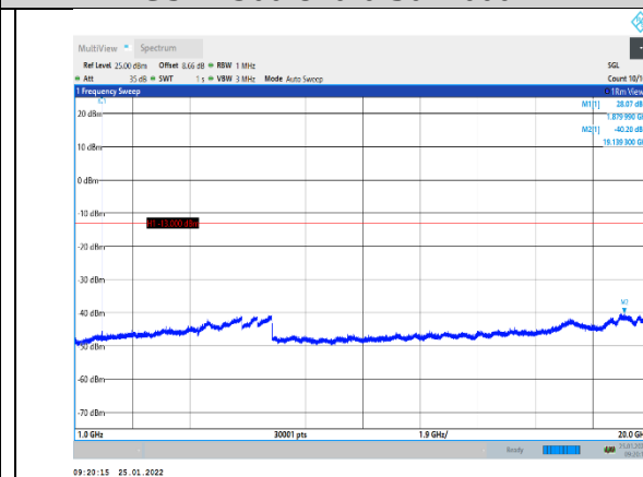
GSM1900-810-0-1000~20000MHz
