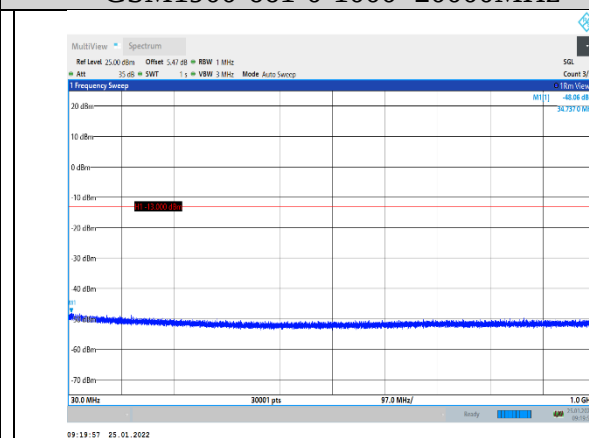
GSM1900-810-0-30~1000MHz
