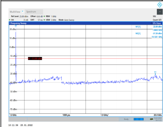
Band2-15MHz-QPSK-18675-1RB#0-Range2: 000~20000MHz
