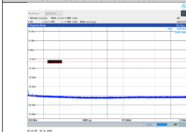
GSM1900-661-0-30~1000MHz
