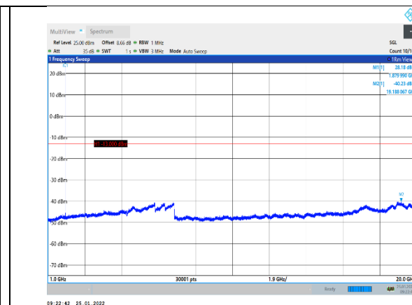
GPRS1900-661-0-1000~20000MHz
