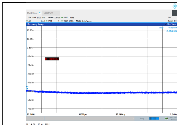
GSM1900-512-0-30~1000MHz
