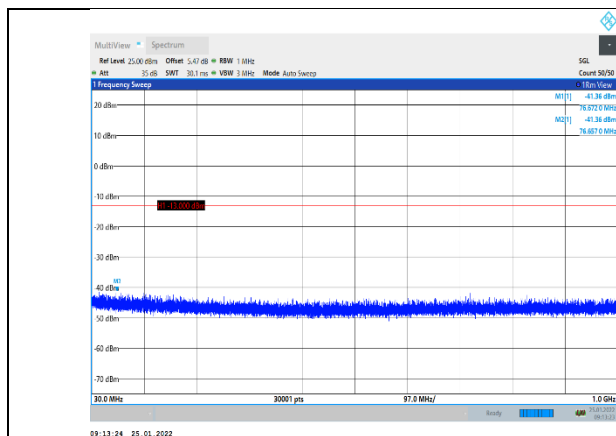
EGPRS850-128-8-30~1000MHz
