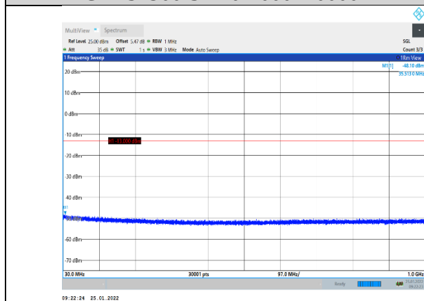
GPRS1900-661-0-30~1000MHz
