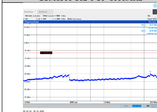
GSM1900-512-0-1000~20000MHz
