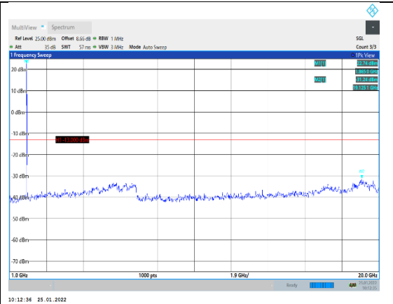
Band2-15MHz-QPSK-18900-1RB#0-Range2: 1 000~20000MHz
