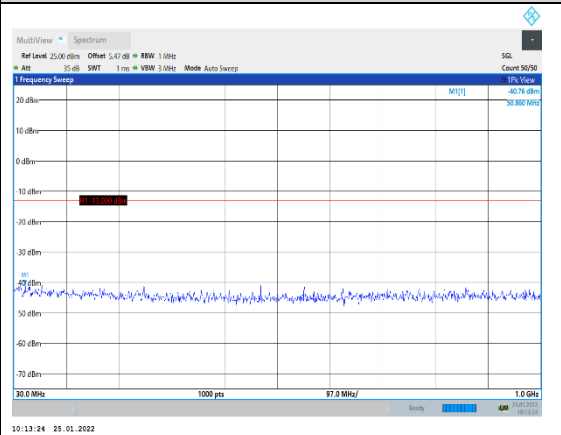
Band2-15MHz-QPSK-19125-1RB#0-Range1:3 0~1000MHz
