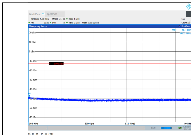
GPRS1900-512-0-30~1000MHz
