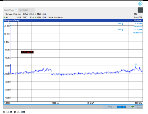
Band2-15MHz-QPSK-19125-1RB#0-Range2: 1 000~20000MHz
