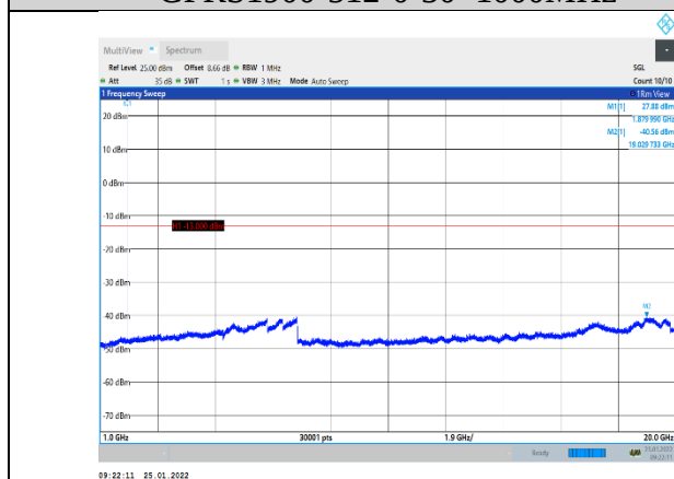
GPRS1900-512-0-1000~20000MHz
