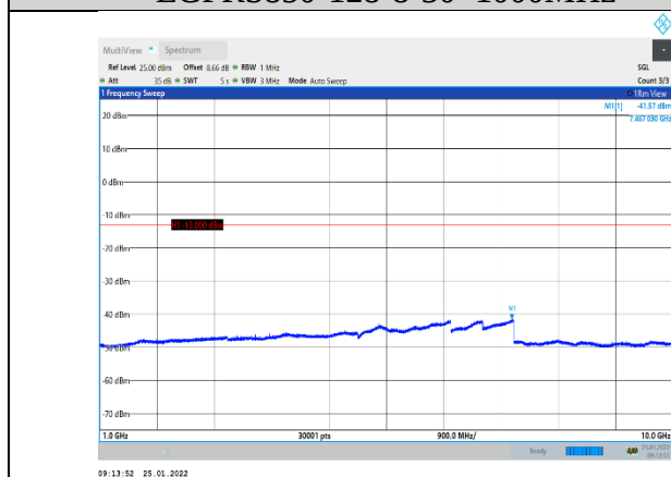
EGPRS850-128-8-1000~10000MHz
