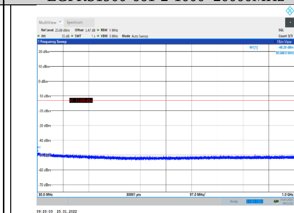
EGPRS1900-810-2-30~1000MHz
