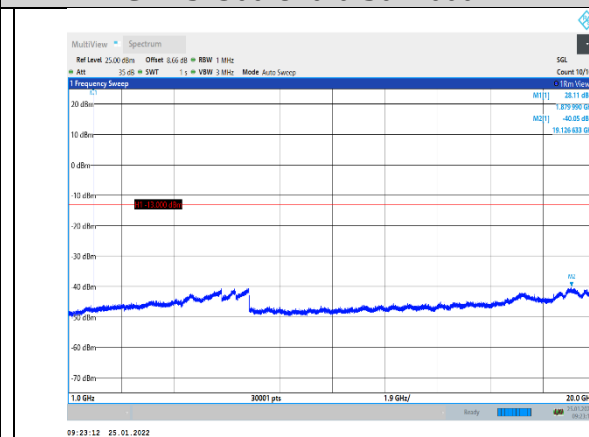
GPRS1900-810-0-1000~20000MHz
