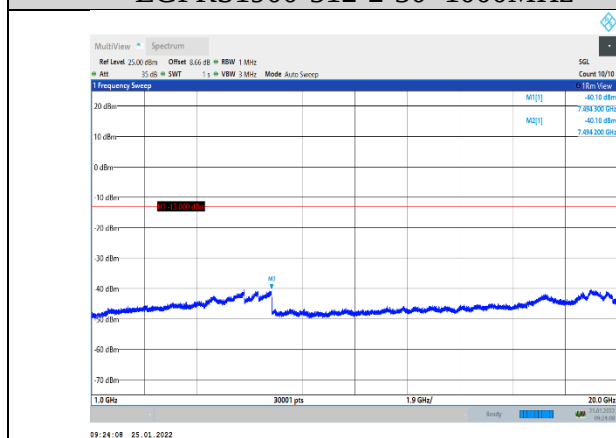
EGPRS1900-512-2-1000~20000MHz
