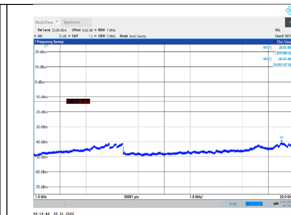
GSM1900-661-0-1000~20000MHz
