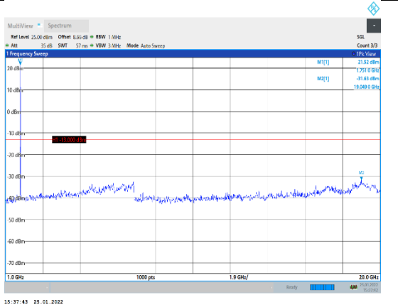
Band4-3MHz-QPSK-20385-1RB#0-Range2:10 00~20000MHz
