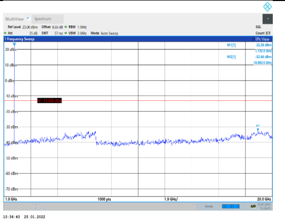
Band4-3MHz-QPSK-20175-1RB#0-Range2:10 00~20000MHz
