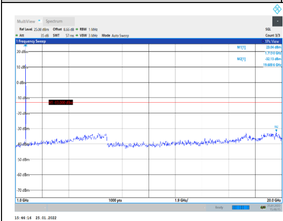
Band4-15MHz-QPSK-20025-1RB#0-Range2: 000~20000MHz
