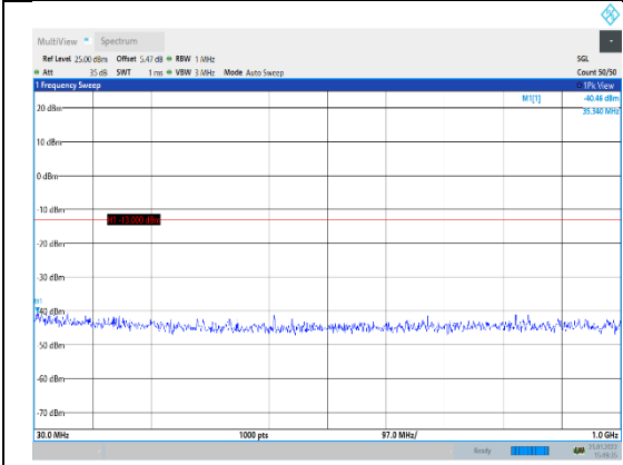
Band4-20MHz-QPSK-20050-1RB#0-Range1: 0~1000MHz
