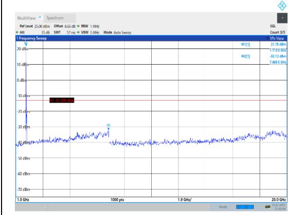
Band4-20MHz-QPSK-20050-1RB#0-Range2: 000~20000MHz
