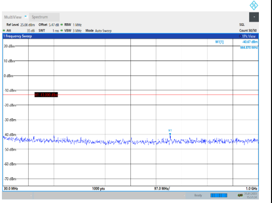
Band4-20MHz-QPSK-20300-1RB#0-Range1:3 0~1000MHz
