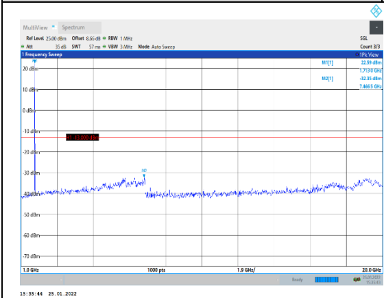
Band4-3MHz-QPSK-19965-1RB#0-Range2:1 00~20000MHz
