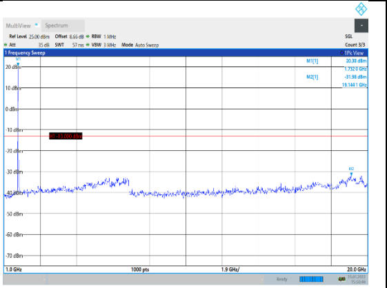
Band4-20MHz-QPSK-20175-1RB#0-Range2:1 000~20000MHz
