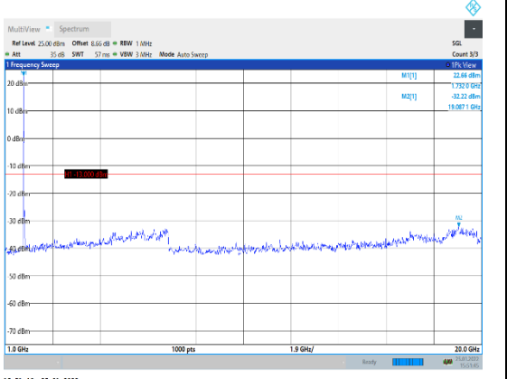
Band4-20MHz-QPSK-20300-1RB#0-Range2:1 000~20000MHz
