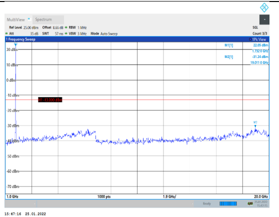
Band4-15MHz-QPSK-20175-1RB#0-Range2:1 000~20000MHz
