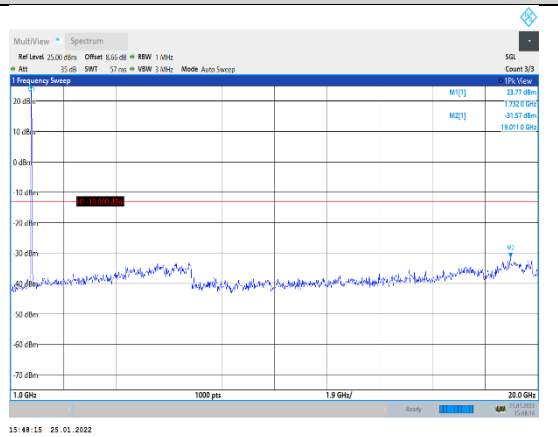
Band4-15MHz-QPSK-20325-1RB#0-Range2:1 000~20000MHz
