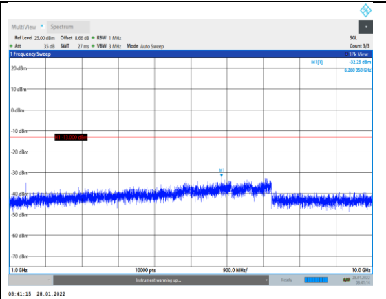
Band12-3MHz-QPSK-23095-1RB#0-Range2:1 000~10000MHz
