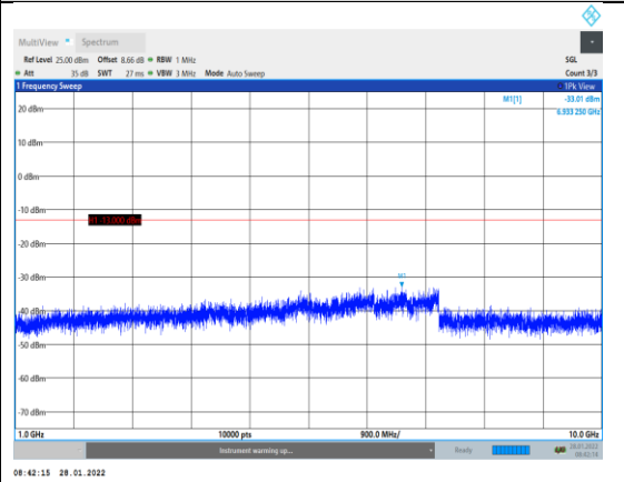
Band12-3MHz-QPSK-23165-1RB#0-Range2:1 000~10000MHz
