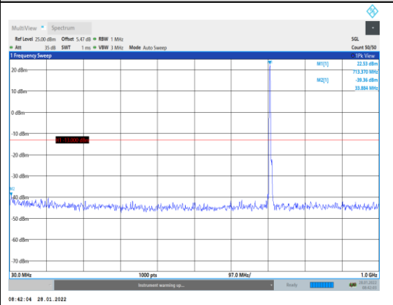
Band12-3MHz-QPSK-23165-1RB#0-Range1:3 0~1000MHz
