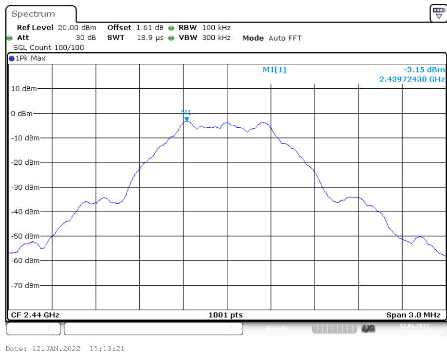
PSD NVNT BLE 1M 2440MHz
