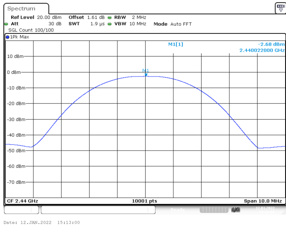
Power NVNT BLE 1M 2440MHz
