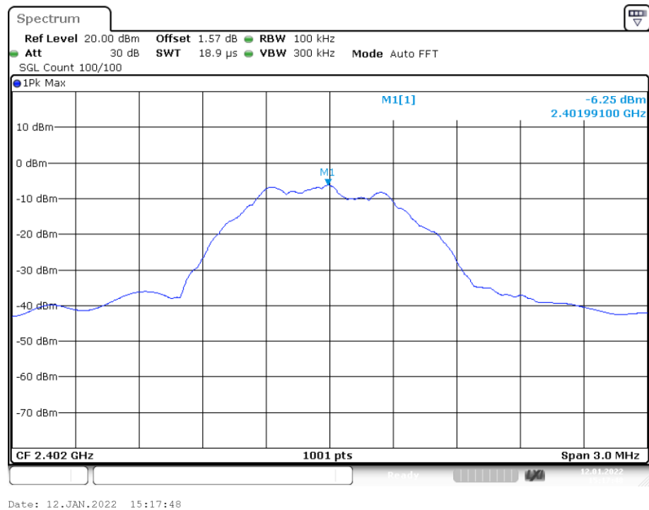
PSD NVNT BLE 1M 2402MHz
