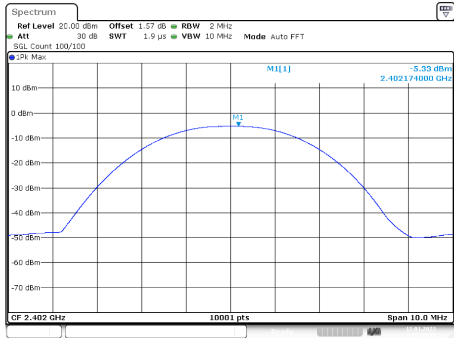
Power NVNT BLE 1M 2402MHz
