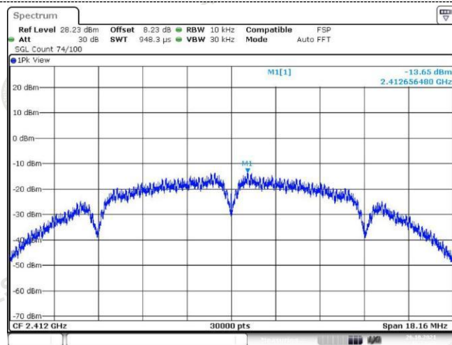
802.11b
