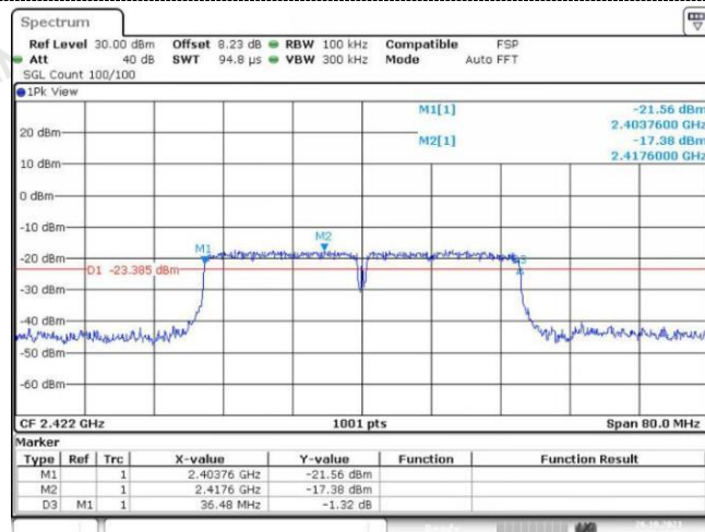
802.11n(HT40)
