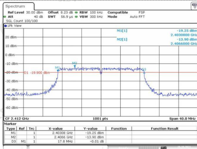
802.11n(HT20)
