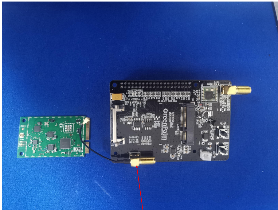
Lora ANT
