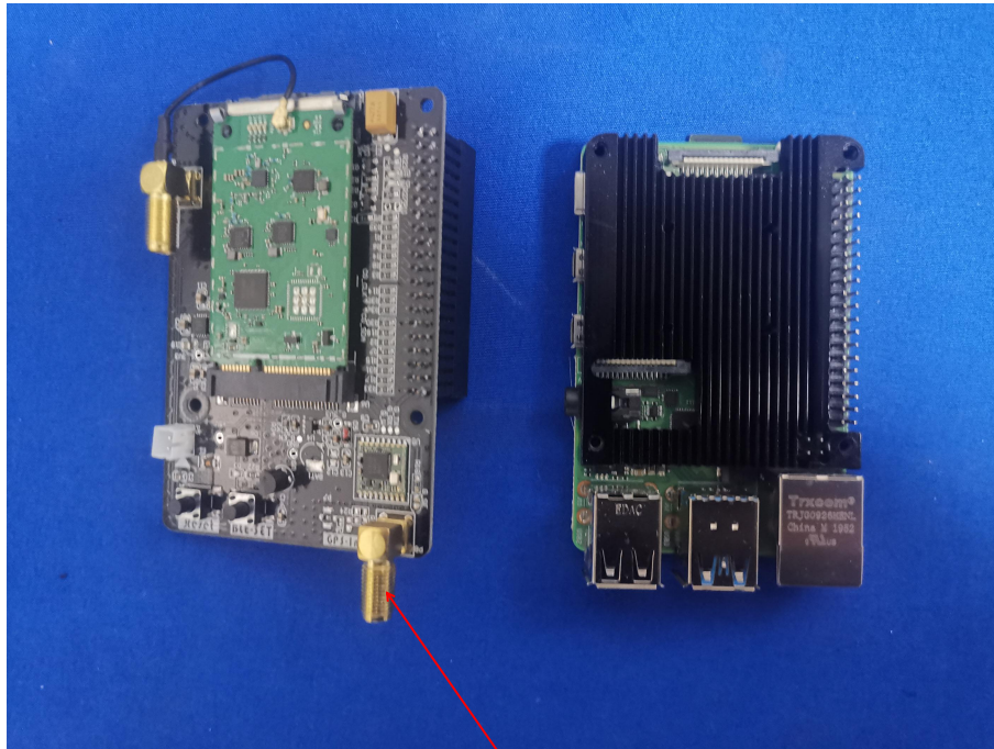
GPS ANT
