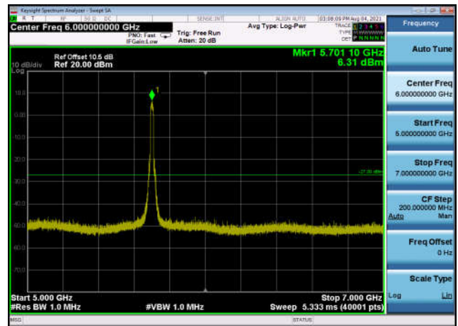
U-NII-2c ,Plot 3,5000MHz~7000MHz-802. 11ac(40MHz),5670MHz,Ant1
