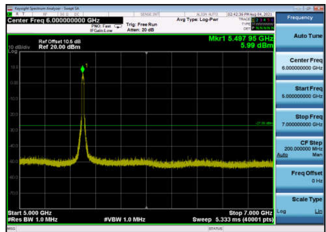
U-NII-2c ,Plot 3,5000MHz~7000MHz-802. 11ac(20MHz),5500MHz,Ant1
