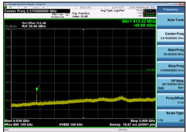
U-NII-2a ,Plot 2,30MHz~5000MHz-802.11 ac(40MHz),5270MHz,Ant1
