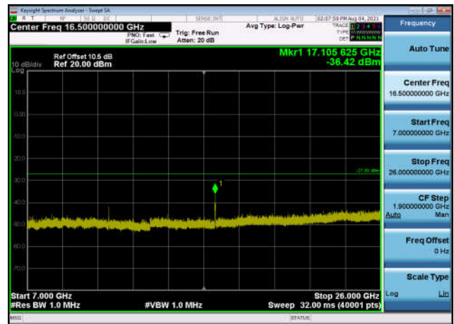
U-NII-2c ,Plot 4,7000MHz~26000MHz-802 .11ac(20MHz),5580MHz,Ant1
