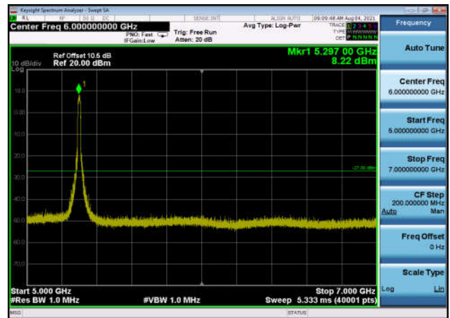
U-NII-2a ,Plot 3,5000MHz~7000MHz-802. 11ac(20MHz),5260MHz,Ant1
