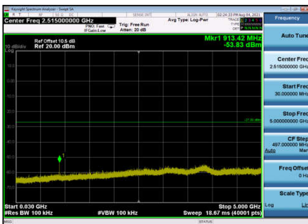
U-NII-2c ,Plot 2,30MHz~5000MHz-802.11 n(20MHz),5580MHz,Ant1
