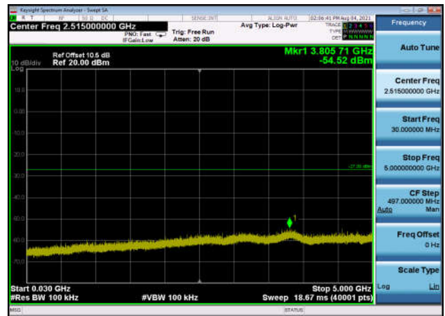
U-NII-2c ,Plot 2,30MHz~5000MHz-802.11 ac(20MHz),5580MHz,Ant1
