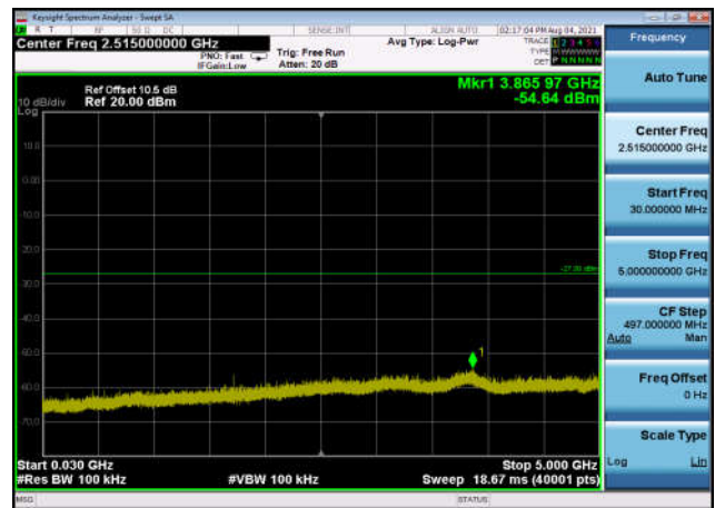
U-NII-2c ,Plot 2,30MHz~5000MHz-802.11 n(20MHz),5700MHz,Ant1
