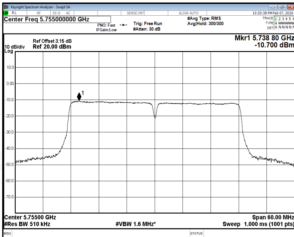
PSD NVNT n40 5755MHz Ant2
