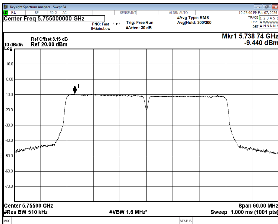
PSD NVNT ax40 5755MHz Ant2
