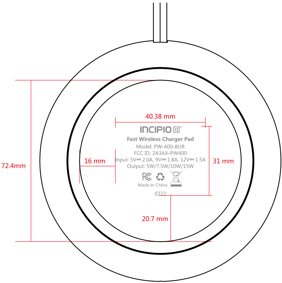
上下左右居中 LOGO CENTERED E/W AND N/S
