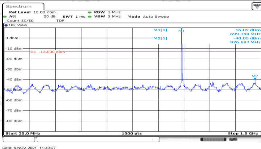
Band12-1.4MHz-QPSK-23017-1RB#0-Range2:1000~10000MHz
