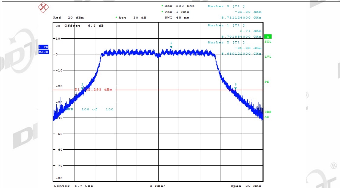
-26dB Bandwidth NVNT a 5700MHz Ant2
