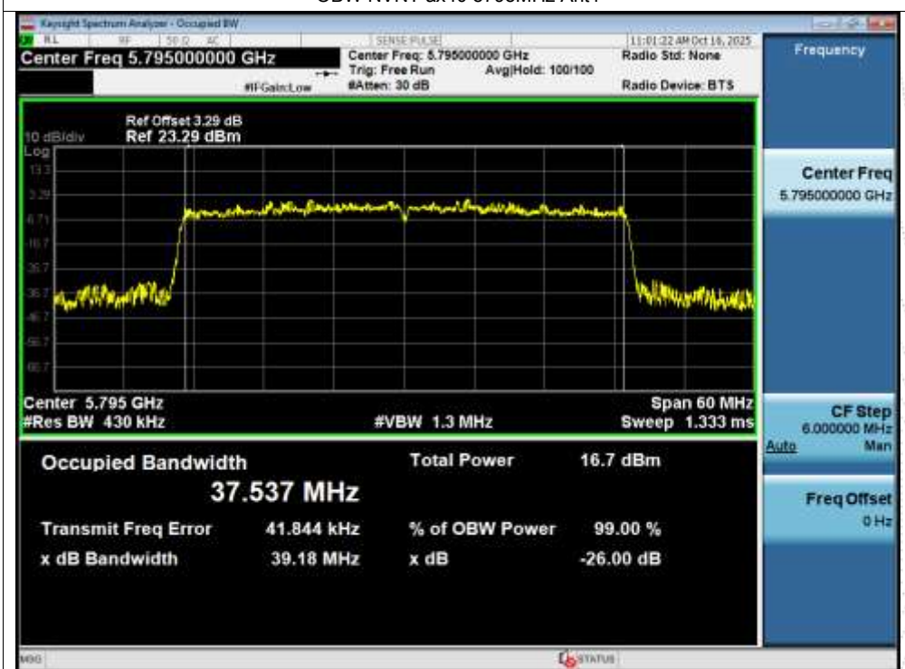
OBW NVNT ax40 5795MHz Ant1
