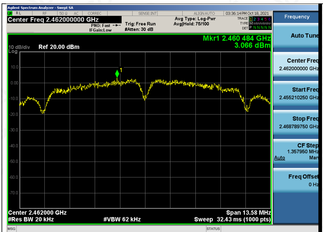
Test_Graph_802.11b_ANT1_2462_1Mbps_PSD
