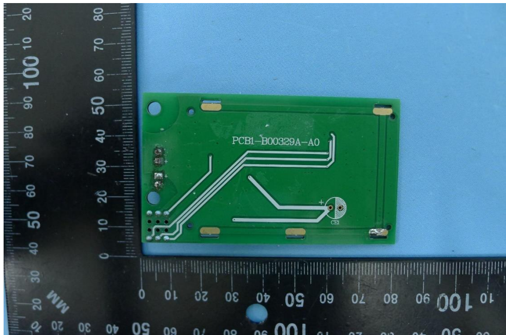
(14) EUT Photo
