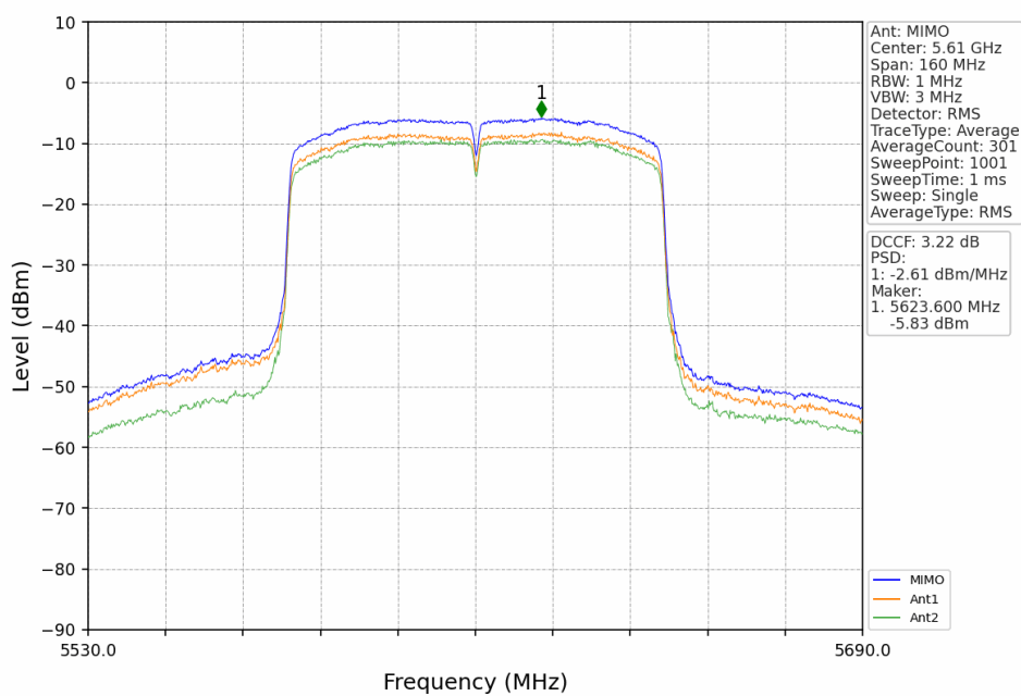
802.11ac(VHT80)_HCH_5610MHz_MIMO_NTNV
