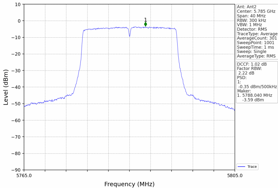
802.11n(HT20)_MCH_5785MHz_MIMO_NTNV
