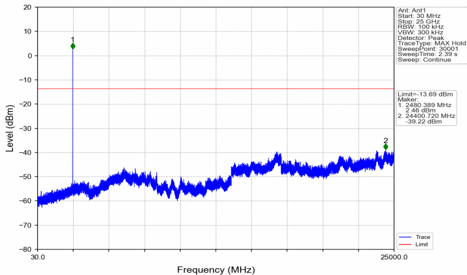
2M_HCH_2480MHz_Ant1_NTNV
