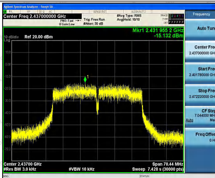
11N40_Ant2_2437
