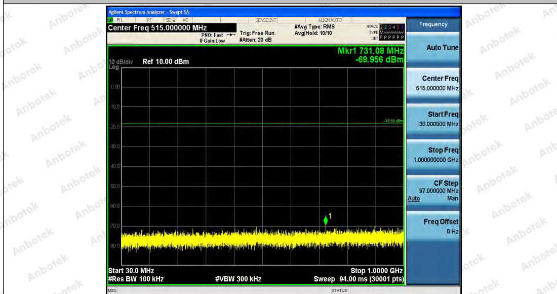
11G_Ant1_2412_30~1000
