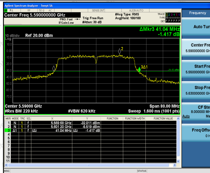
11N40ISO_Ant2_5590
