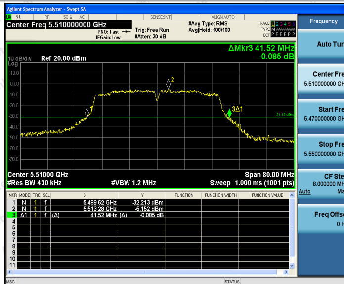
11N40SISO_Ant2_5510
