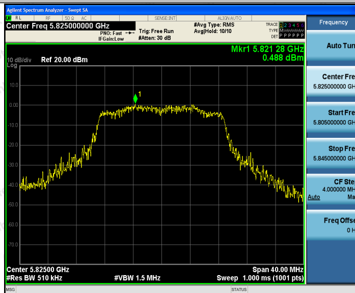
11N20SISO_Ant2_5825
