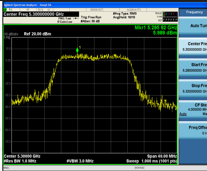
11N20SISO_Ant2_5300
