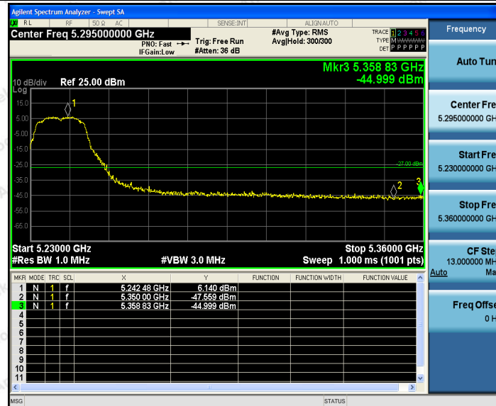
11A_Ant1_Low_5260
