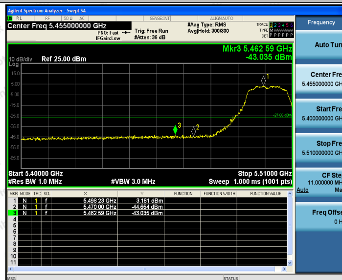
11A_Ant2_Low_5500
