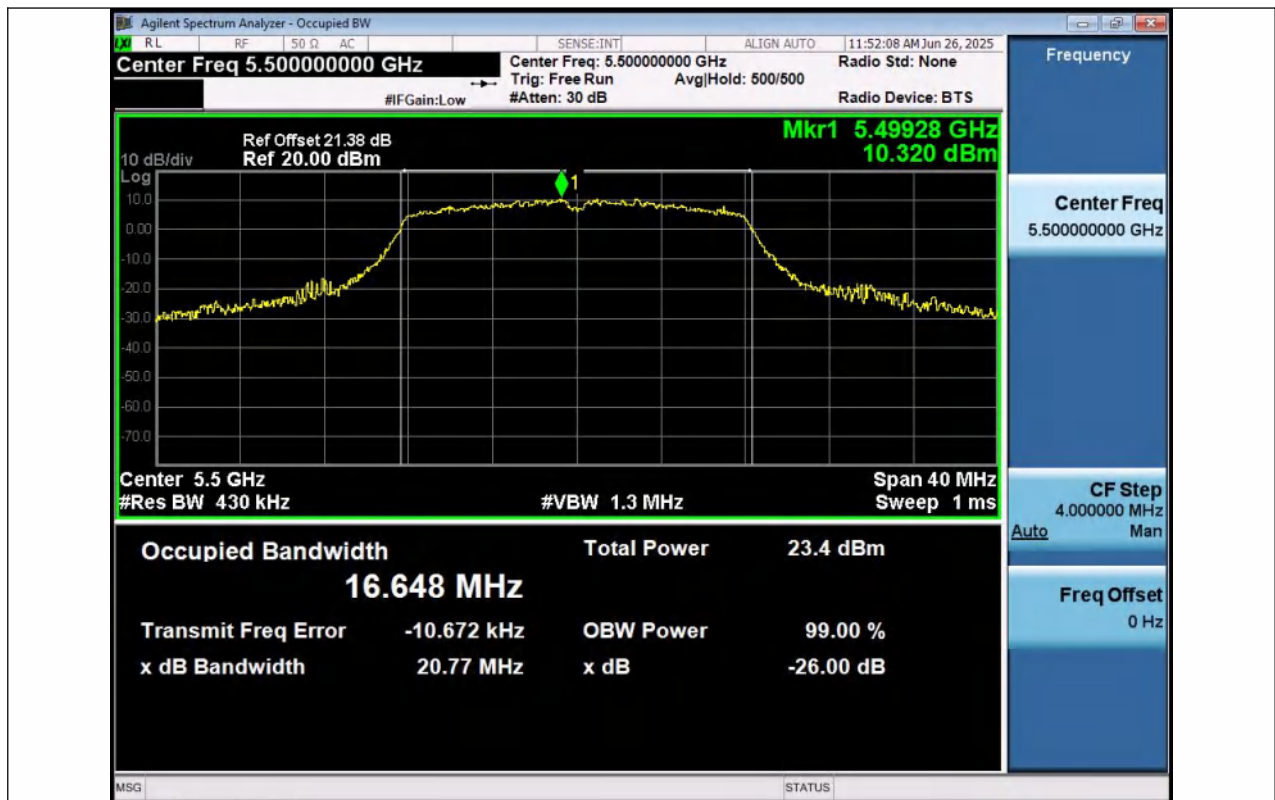
11A-Ant1-5500
