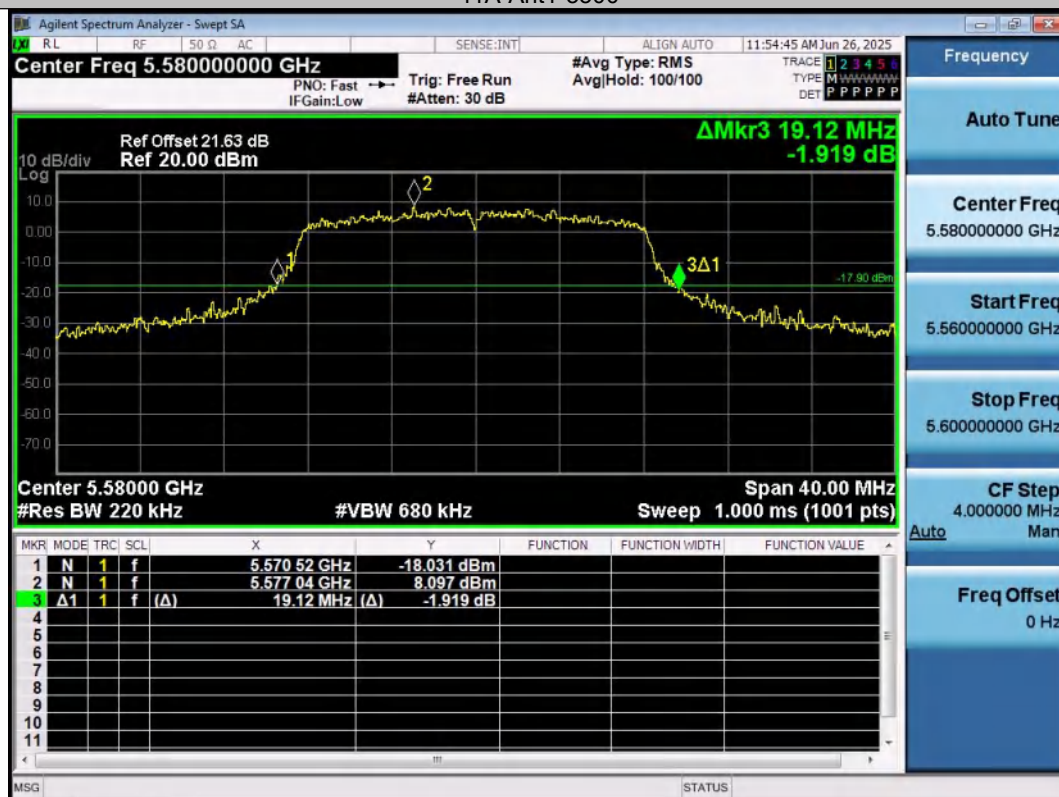
11A-Ant1-5580
