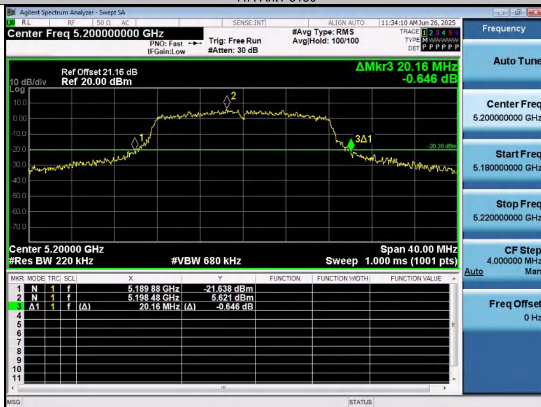
11A-Ant1-5200
