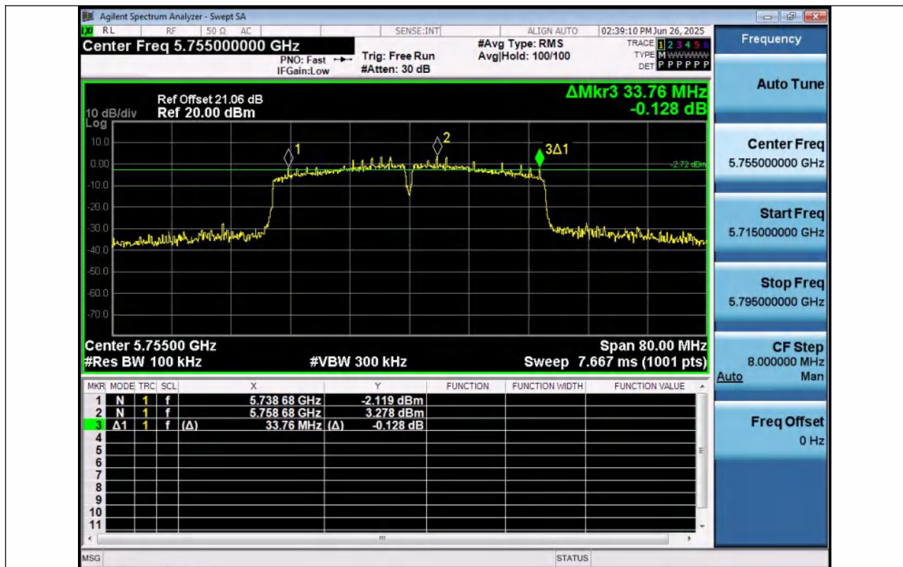
11N40SISO-Ant1-5755-PASS
