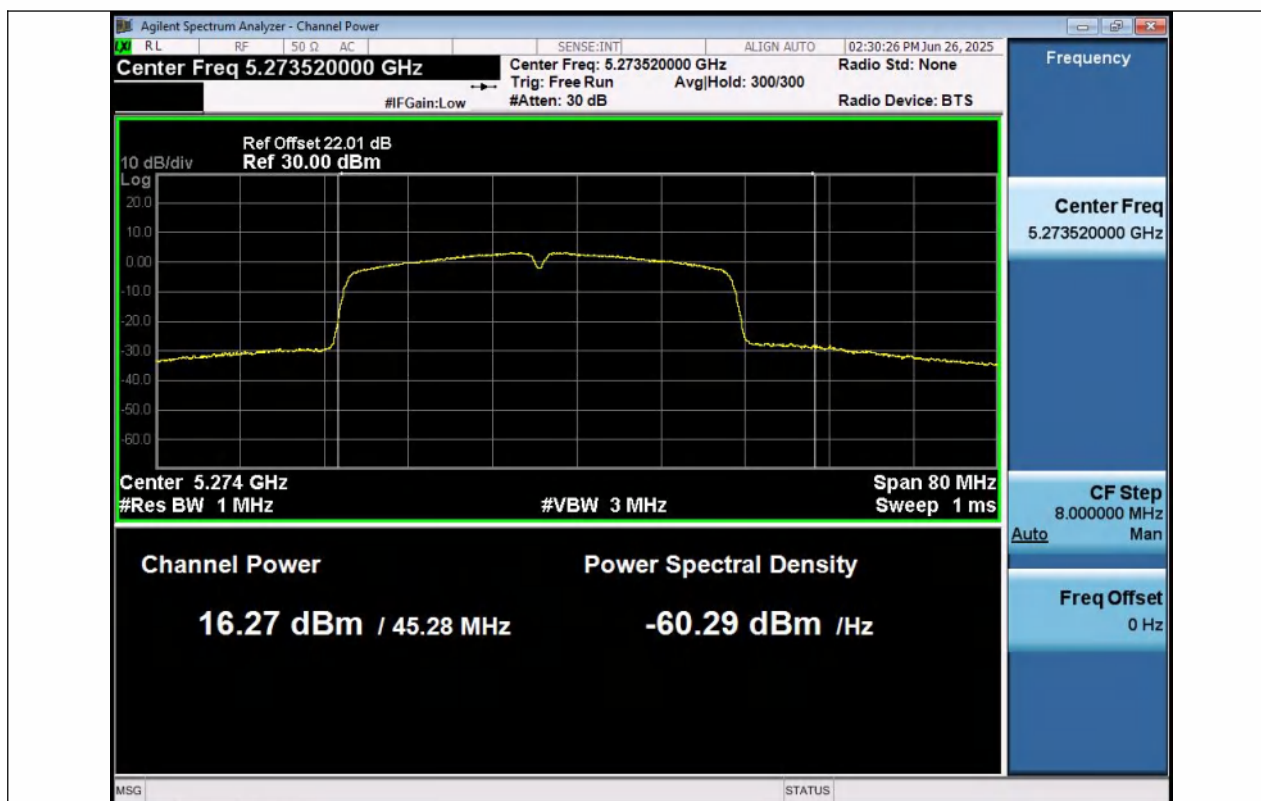
11N40SISO-Ant1-5270-PASS
