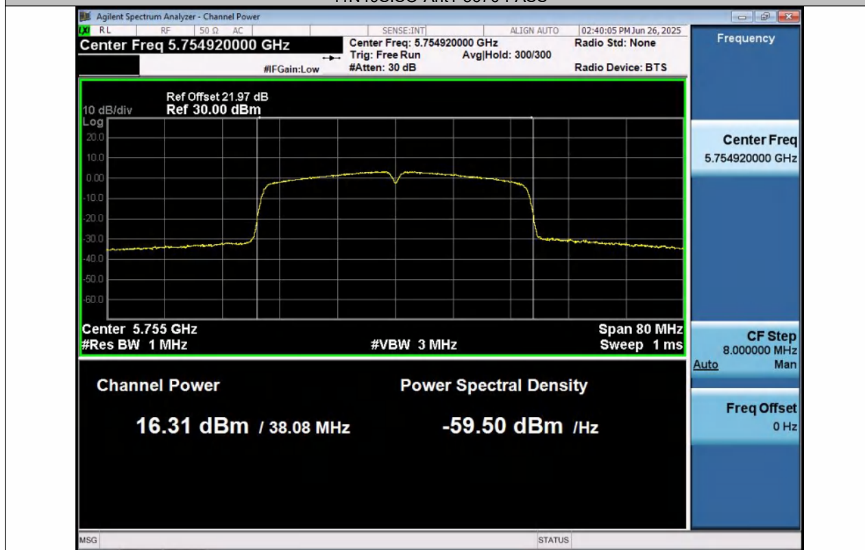
11N40SISO-Ant1-5755-PASS
