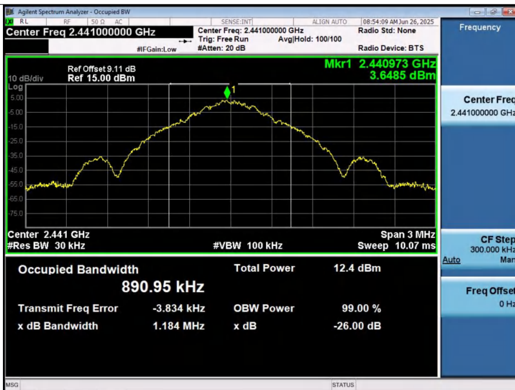
DH5-Ant1-2441
