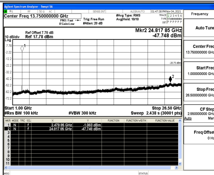
BLE_1M_Ant2_2480_1000~26500
