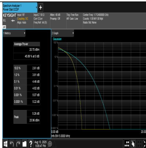
Band4-1312-1-PASS
