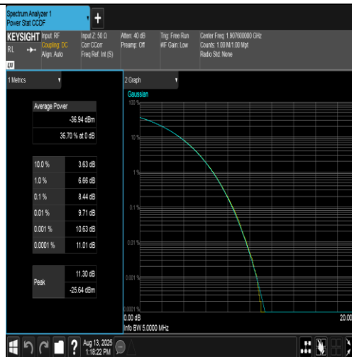
Band2-9538-3-PASS
