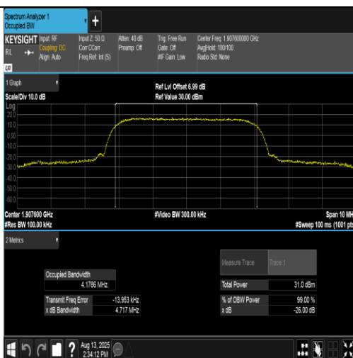
Band2-9538-3-PASS
