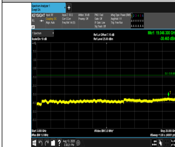
Band4-1513-3000~20000MHz-PASS
