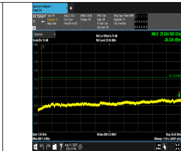
Band4-1513-1000~30000MHz-PASS
