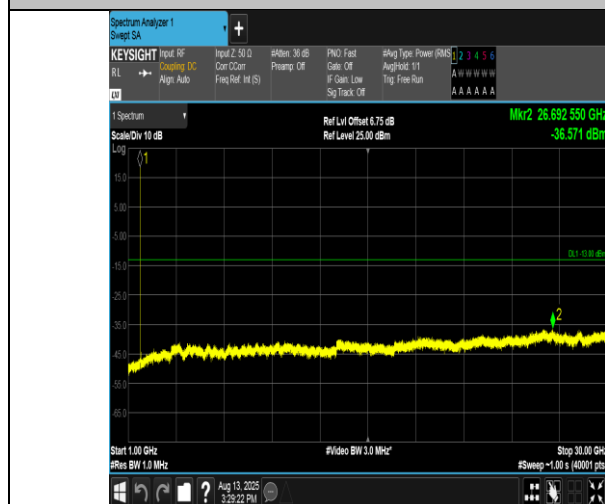
Band4-1413-1000~30000MHz-PASS
