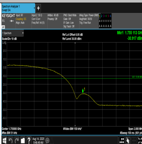
Band4-1513-5-PASS
