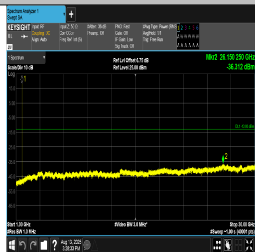
Band4-1312-1000~30000MHz-PASS
