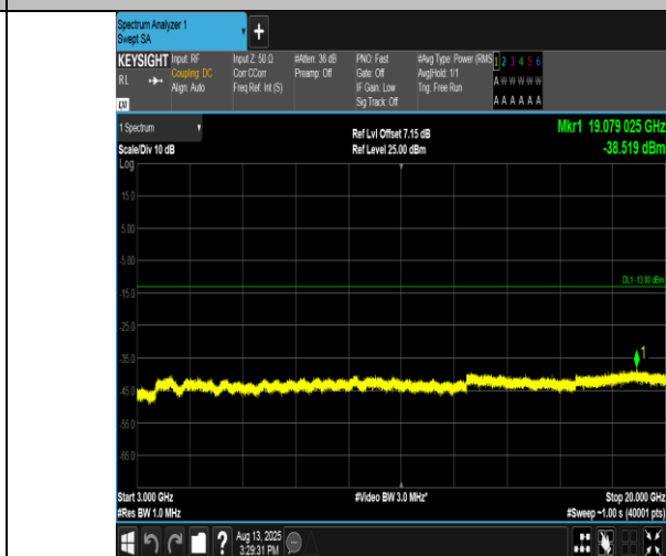
Band4-1413-3000~20000MHz-PASS
