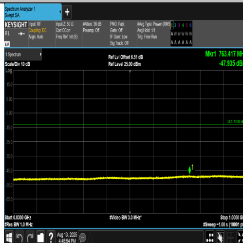
Band4-1312-4-30~1000MHz-PASS
