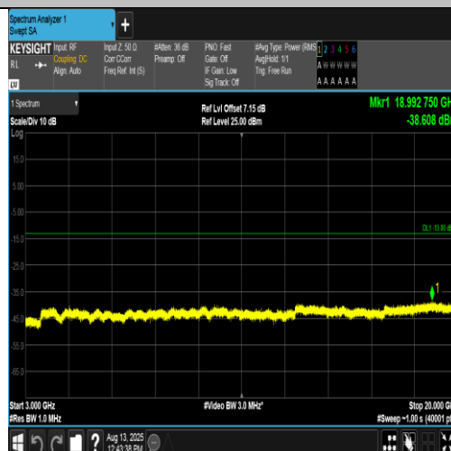
Band2-9538-1-3000~20000MHz-PASS
