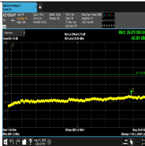
Band4-1312-1-1000~30000MHz-PASS
