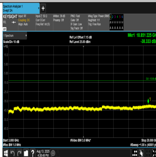
Band4-1312-1-3000~20000MHz-PASS
