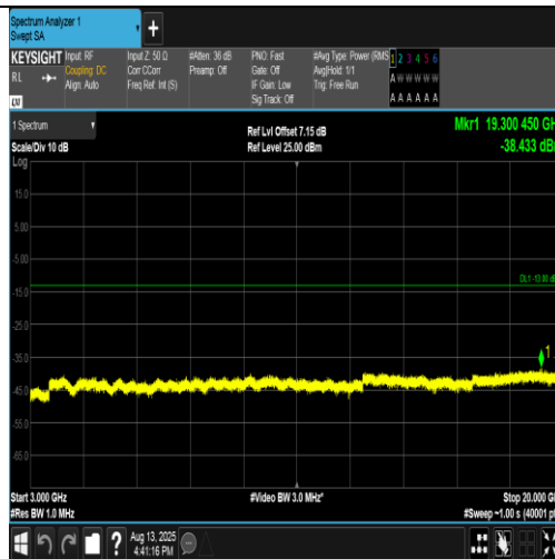
Band4-1312-2-3000~20000MHz-PASS
