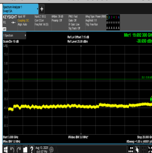
Band4-1413-2-3000~20000MHz-PASS
