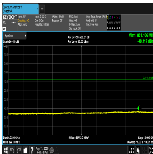
Band4-1413-2-30~1000MHz-PASS
