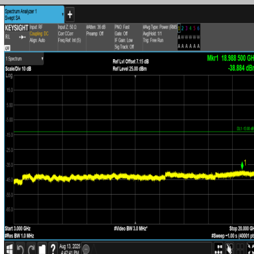
Band4-1513-2-3000~20000MHz-PASS
