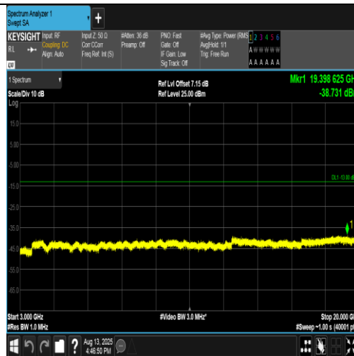
Band4-1413-4-3000~20000MHz-PASS
