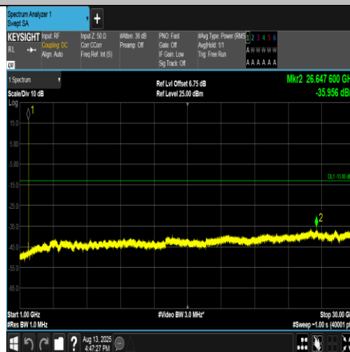
Band4-1513-4-1000~30000MHz-PASS
