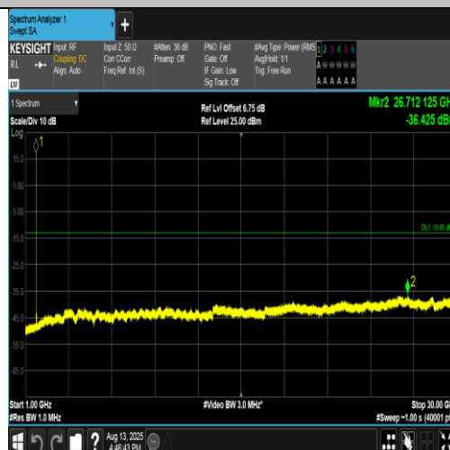
Band4-1413-4-1000~30000MHz-PASS
