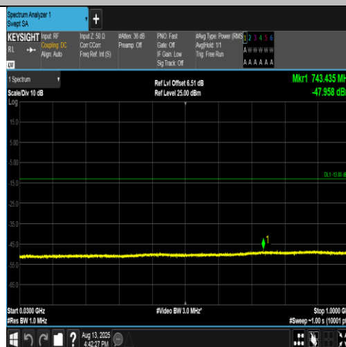
Band4-1513-2-30~1000MHz-PASS
