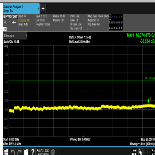
Band4-1513-4-3000~20000MHz-PASS
