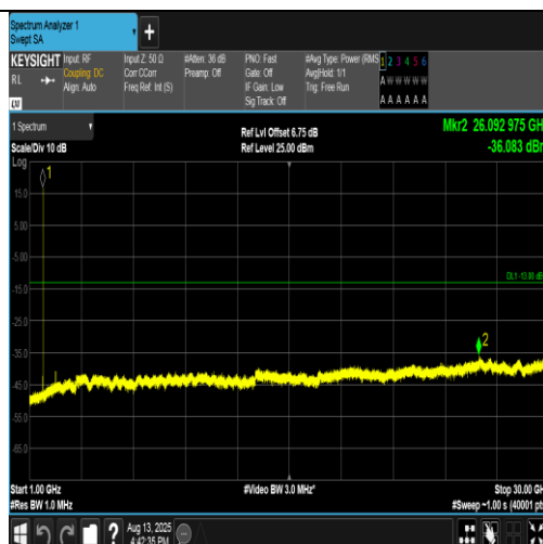
Band4-1513-2-1000~30000MHz-PASS
