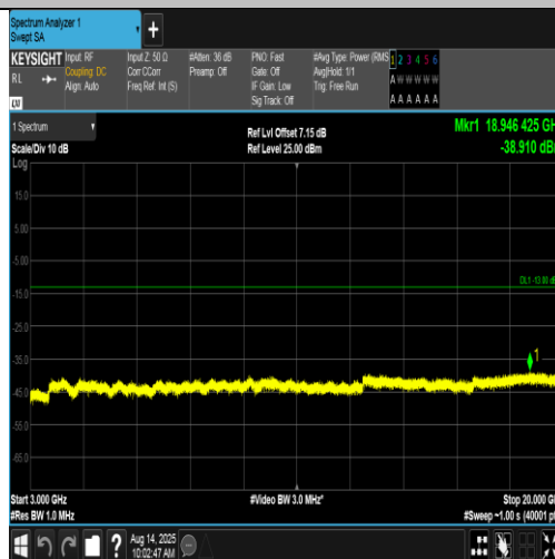
Band4-1312-4-3000~20000MHz-PASS
