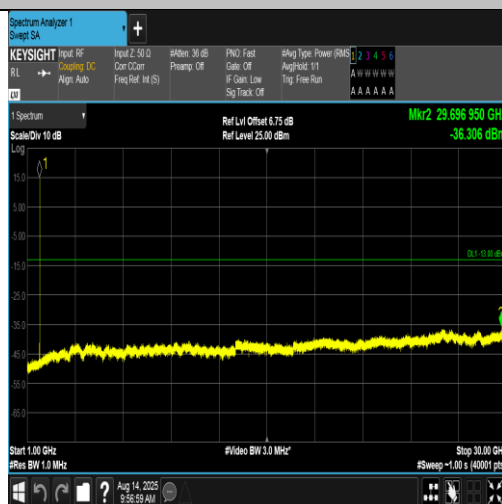
Band4-1513-2-1000~30000MHz-PASS
