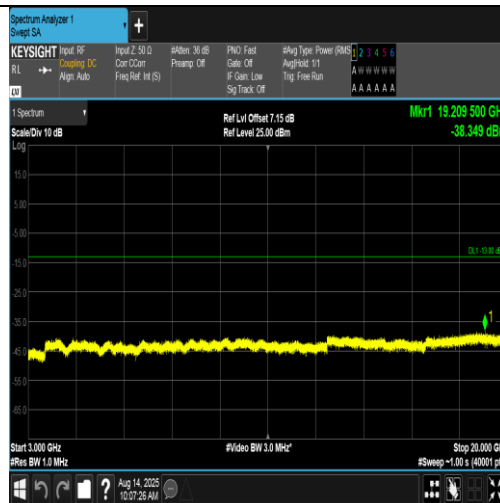
Band4-1312-5-3000~20000MHz-PASS
