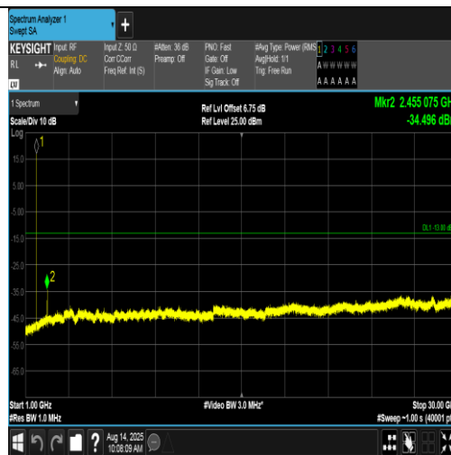
Band4-1413-5-1000~30000MHz-PASS
