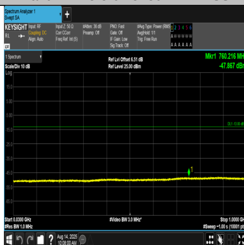
Band4-1413-5-30~1000MHz-PASS
