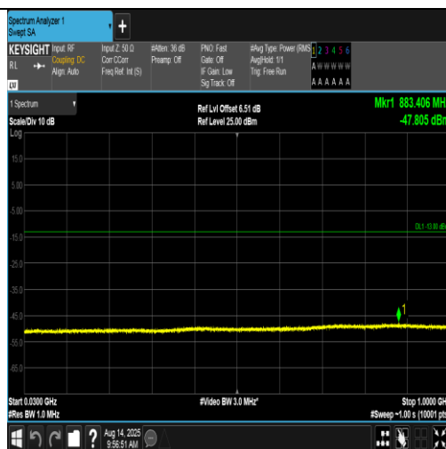
Band4-1513-2-30~1000MHz-PASS
