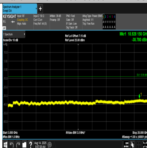
Band4-1513-2-3000~20000MHz-PASS
