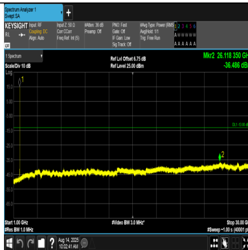
Band4-1312-4-1000~30000MHz-PASS
