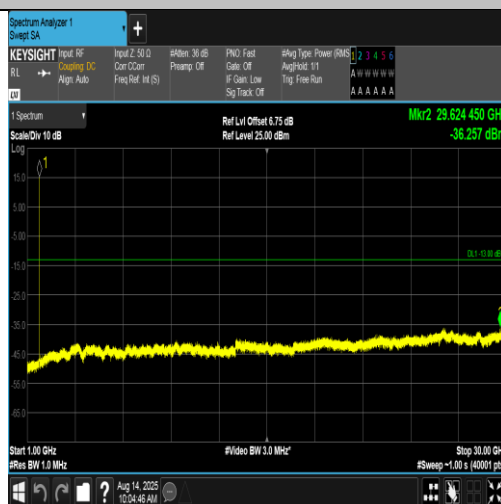
Band4-1413-4-1000~30000MHz-PASS
