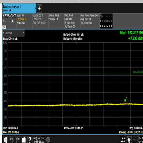
Band4-1413-2-30~1000MHz-PASS
