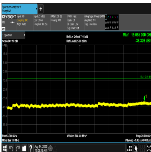
Band4-1513-4-3000~20000MHz-PASS
