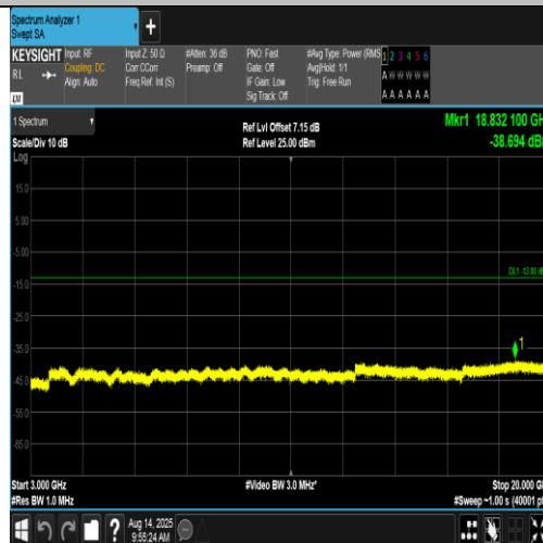
Band4-1413-2-3000~20000MHz-PASS
