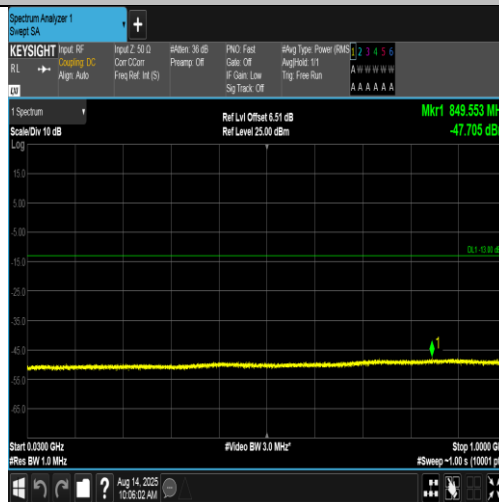
Band4-1513-4-30~1000MHz-PASS
