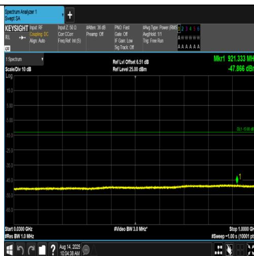
Band4-1413-4-30~1000MHz-PASS
