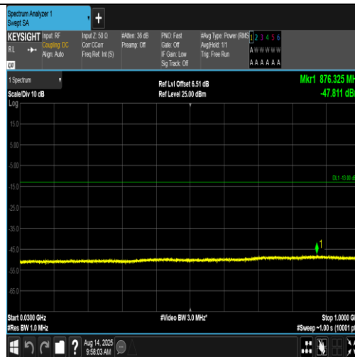
Band4-1312-3-30~1000MHz-PASS
