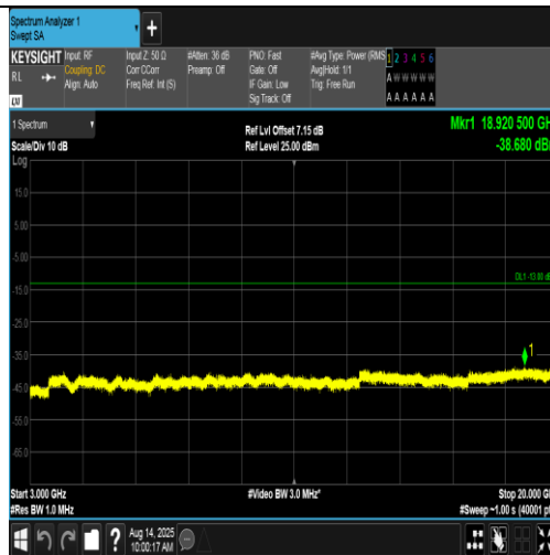
Band4-1413-3-3000~20000MHz-PASS
