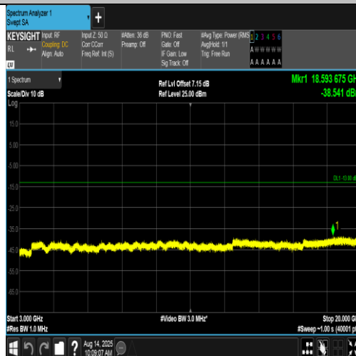
Band4-1513-5-3000~20000MHz-PASS
