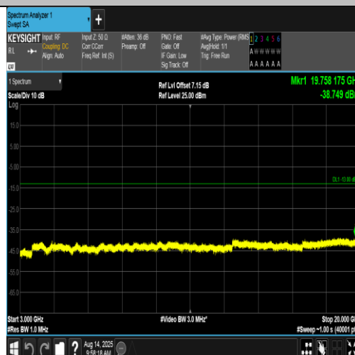
Band4-1312-3-3000~20000MHz-PASS
