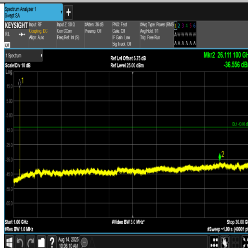
Band4-1513-4-1000~30000MHz-PASS
