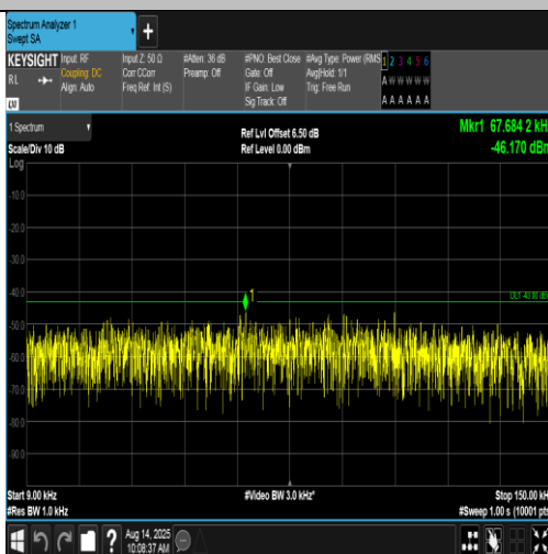
Band4-1513-5-0.009~0.15MHz-PASS
