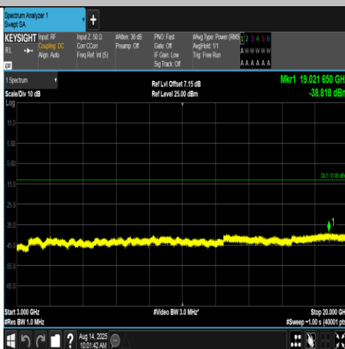
Band4-1513-3-3000~20000MHz-PASS
