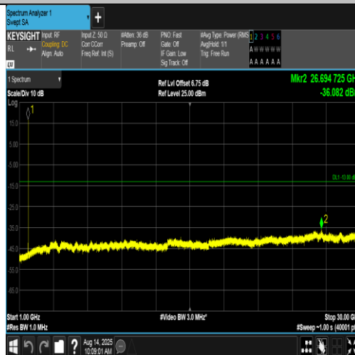
Band4-1513-5-1000~30000MHz-PASS
