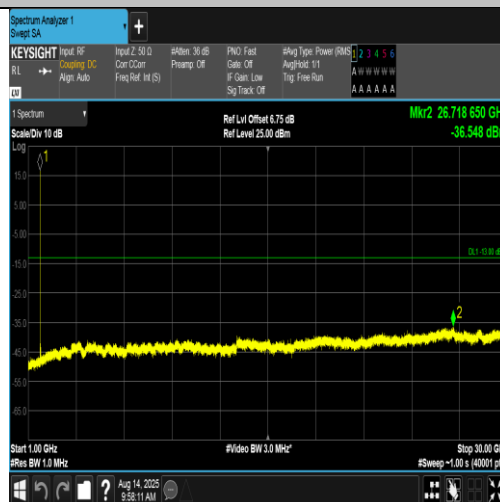
Band4-1312-3-1000~30000MHz-PASS
