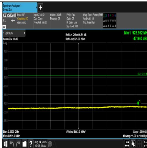
Band4-1513-5-30~1000MHz-PASS
