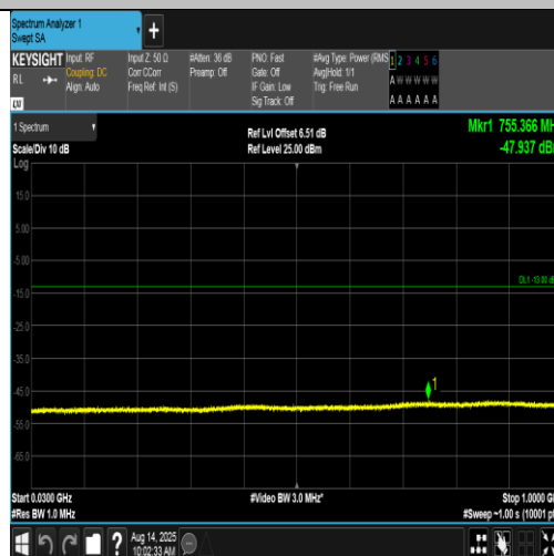
Band4-1312-4-30~1000MHz-PASS
