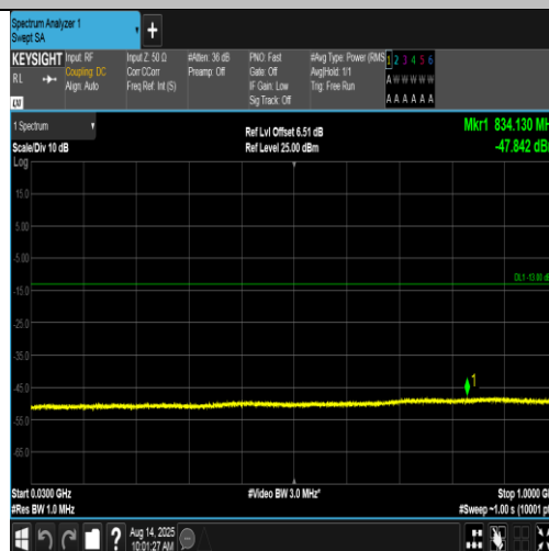
Band4-1513-3-30~1000MHz-PASS
