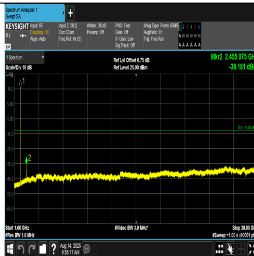
Band4-1413-2-1000~30000MHz-PASS
