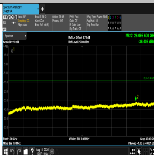
Band4-1312-5-1000~30000MHz-PASS
