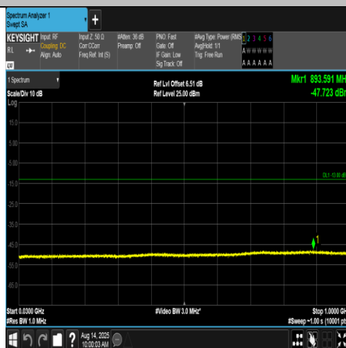
Band4-1413-3-30~1000MHz-PASS
