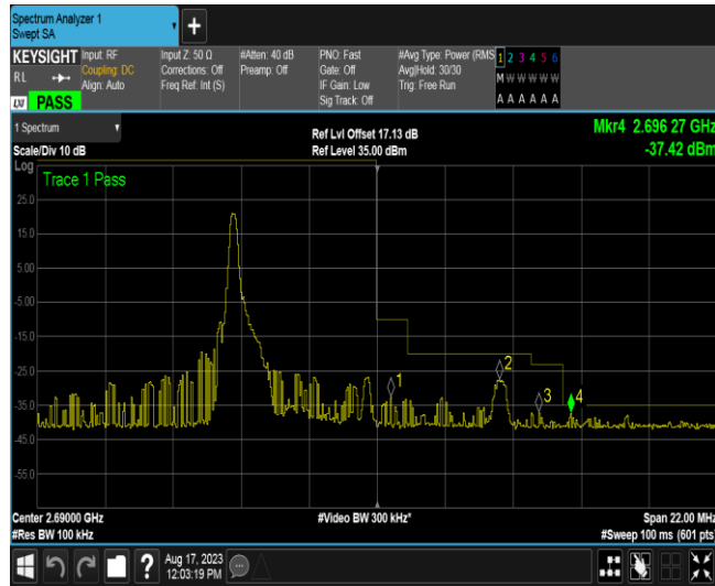
Band41-5MHz-16QAM-41565-1RB#24
