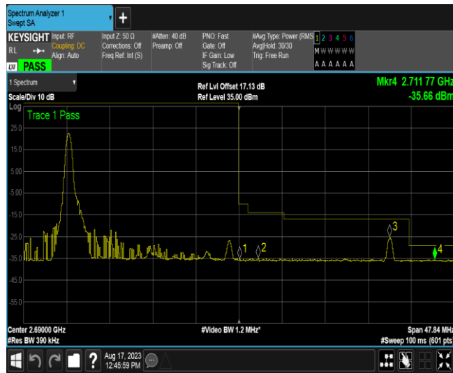
Band41-20MHz-QPSK-41490-1RB#99
