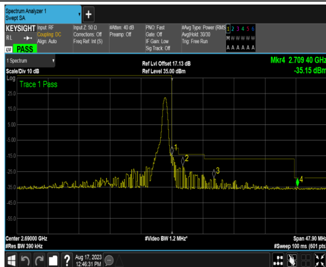
Band41-20MHz-16QAM-41490-1RB#99
