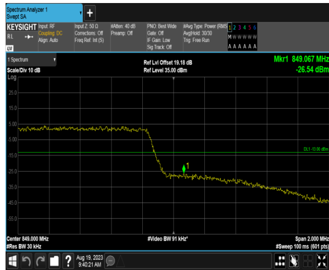
Band5-3MHz-QPSK-20415-1RB#0
