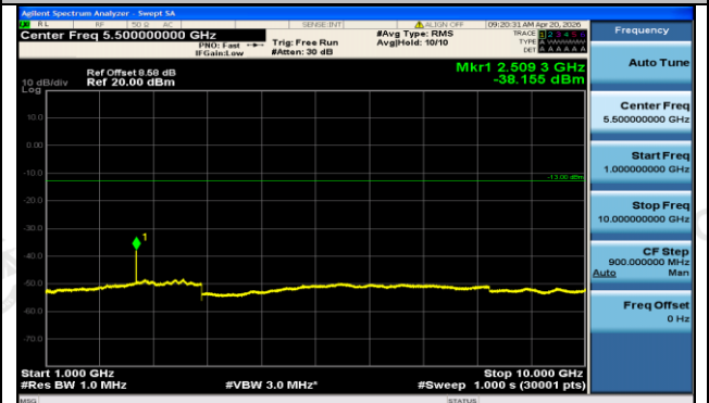
GSM850-190-5-1000~10000MHz-PASS
