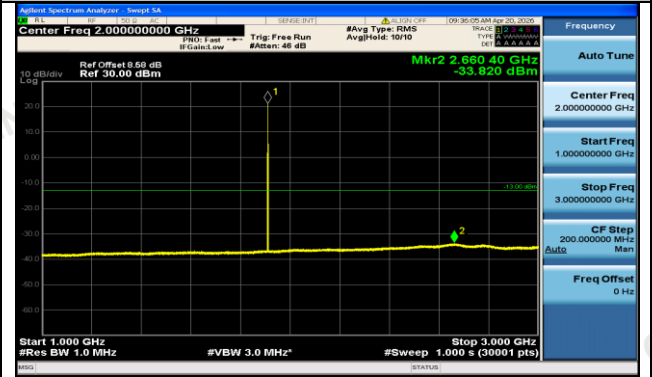
GSM1900-810-0-1000~3000MHz-PASS
