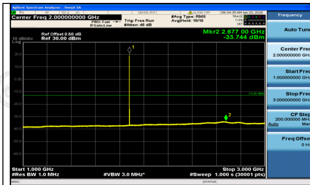
GSM1900-661-0-1000~3000MHz-PASS
