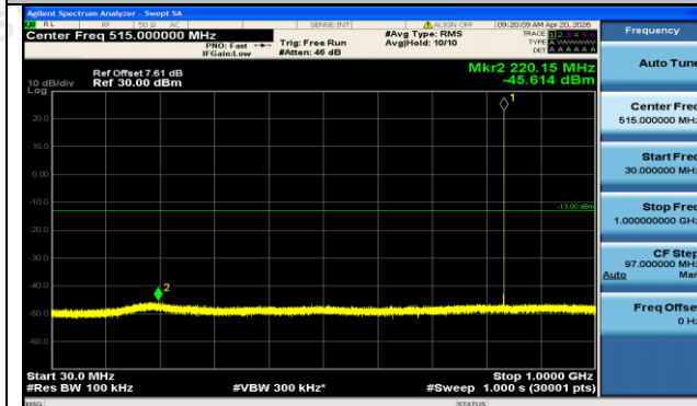
GSM850-190-5-30~1000MHz-PASS
