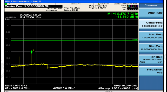
GSM850-128-5-1000~10000MHz-PASS
