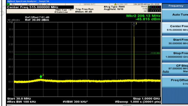
GSM850-128-5-30~1000MHz-PASS
