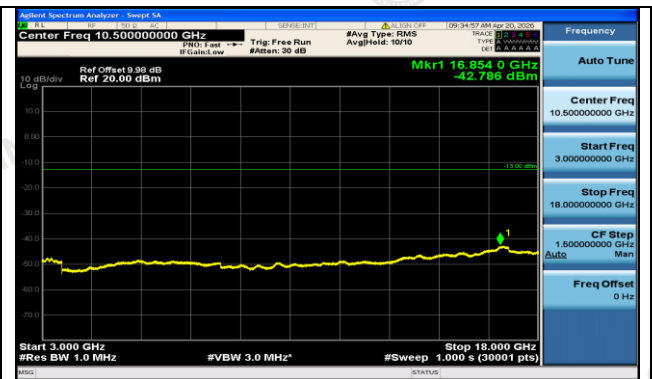
GSM1900-661-0-3000~18000MHz-PASS
