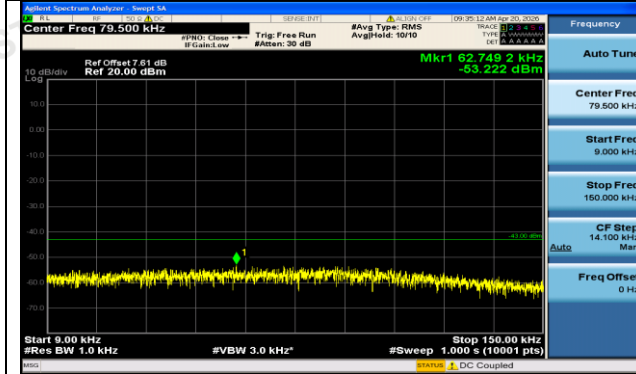
GSM1900-810-0-0.009~0.15MHz-PASS
