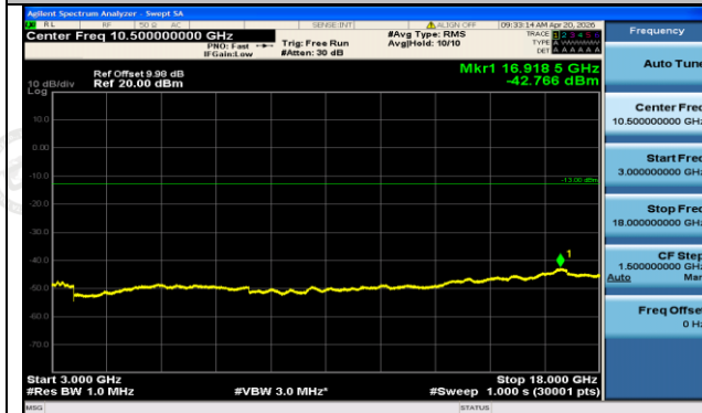
GSM1900-512-0-3000~18000MHz-PASS
