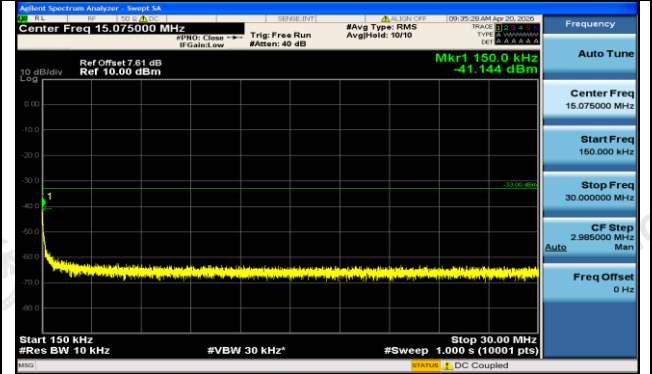
GSM1900-810-0-0.15~30MHz-PASS
