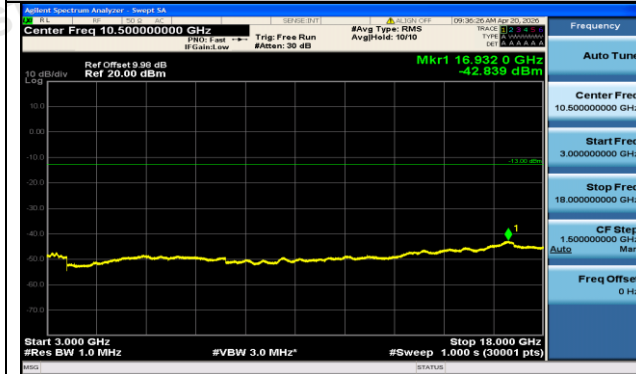
GSM1900-810-0-3000~18000MHz-PASS
