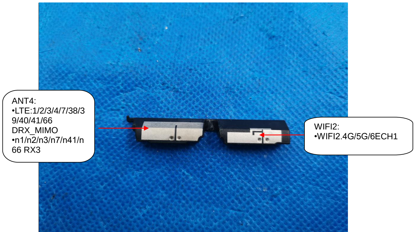
ANT4&WIFI2
