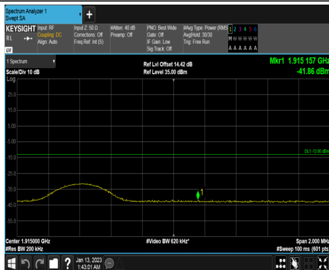
Band25-10MHz-QPSK-26640-1RB#0
