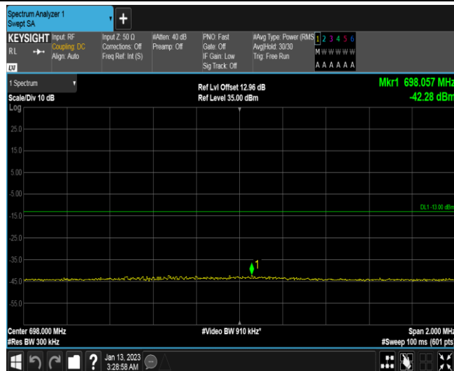
Band71-15MHz-QPSK-133397-1RB#74
