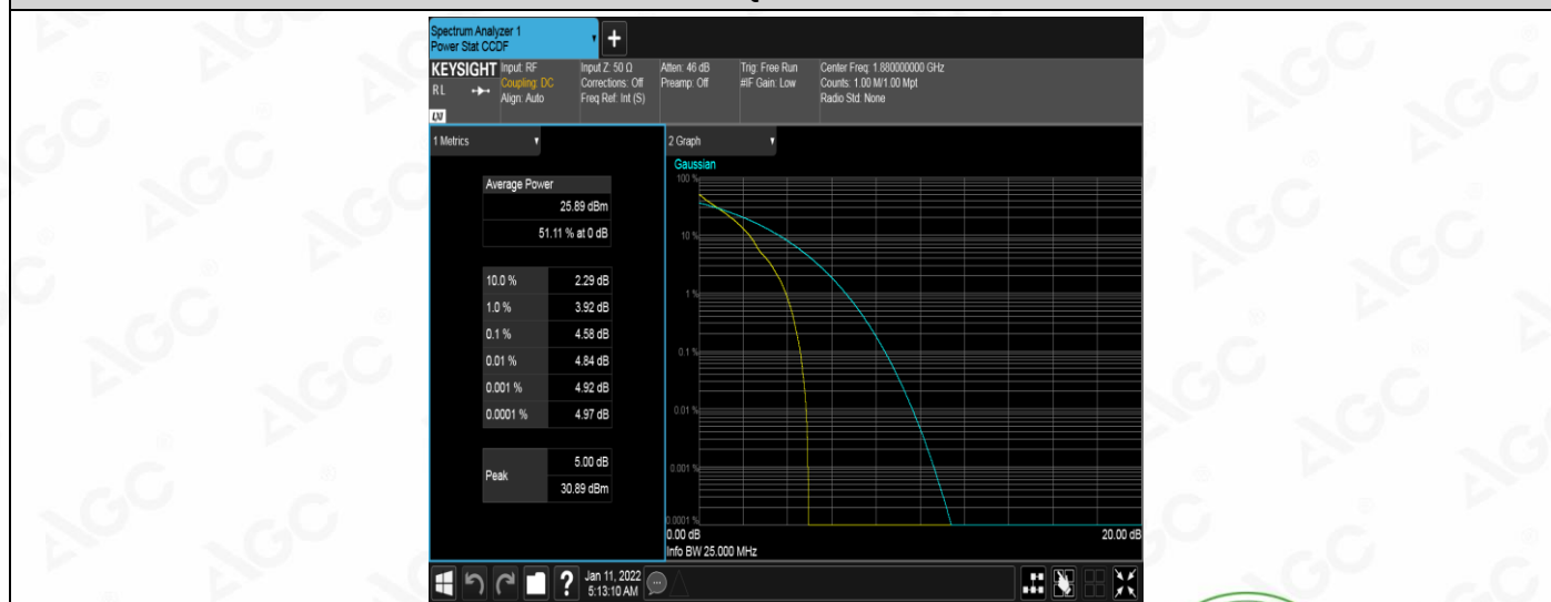
Band2-3MHz-QPSK-18900-1RB#0
