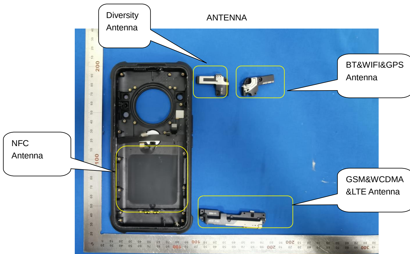
GSM&WCDMA&LTE ANTENNA
