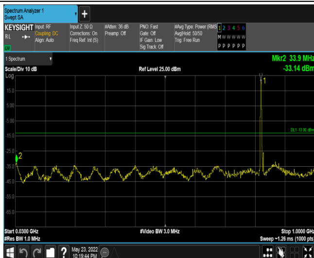
Band5-3MHz-QPSK-20415-1RB#0-Range2:30~1000MHz
