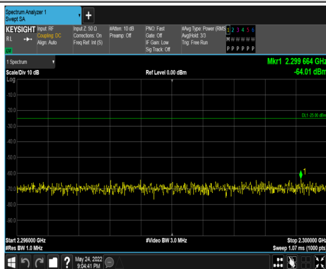
Band40-10MHz-QPSK-38750-1RB#0-Range5:2296~2300MHz
