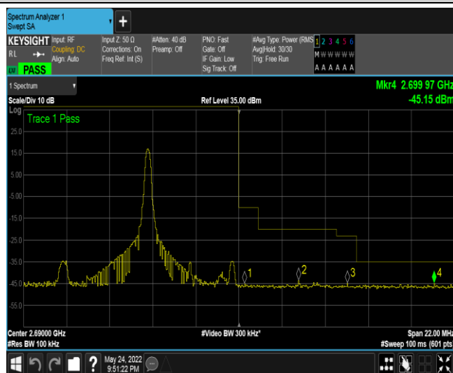
Band41-5MHz-QPSK-41565-1RB#0
