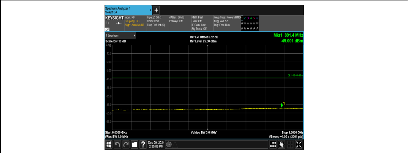
Band2-9538-3-30~1000MHz-PASS
