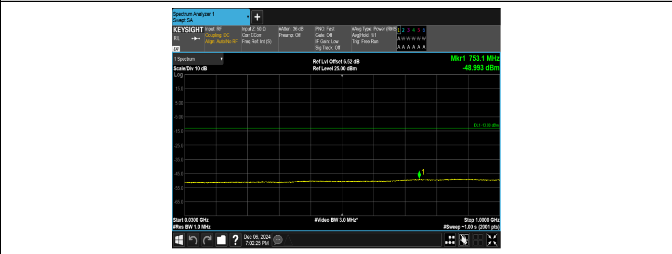
Band4-1312-1-30~1000MHz-PASS
