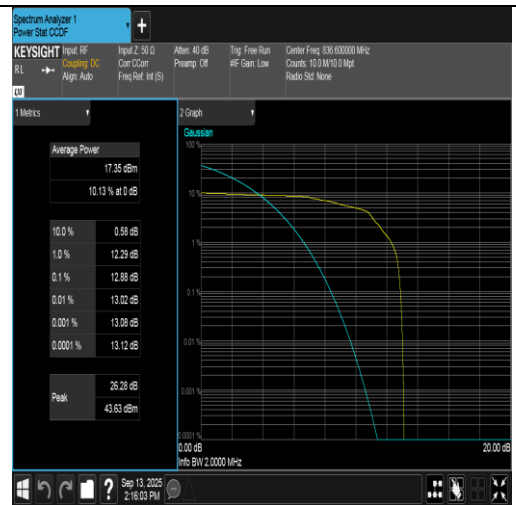
EGPRS850-190-8-PASS
