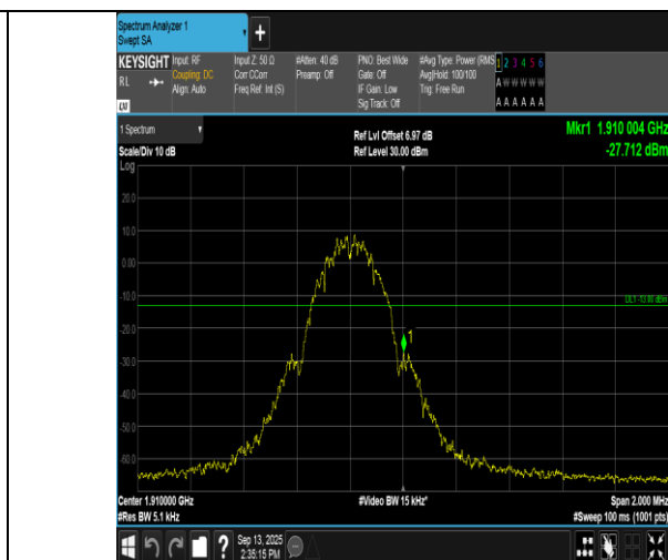
GSM1900-810-0-PASS
