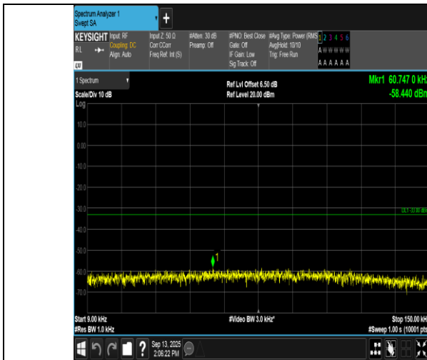
GPRS850-128-5-0.009~0.15MHz-PASS
