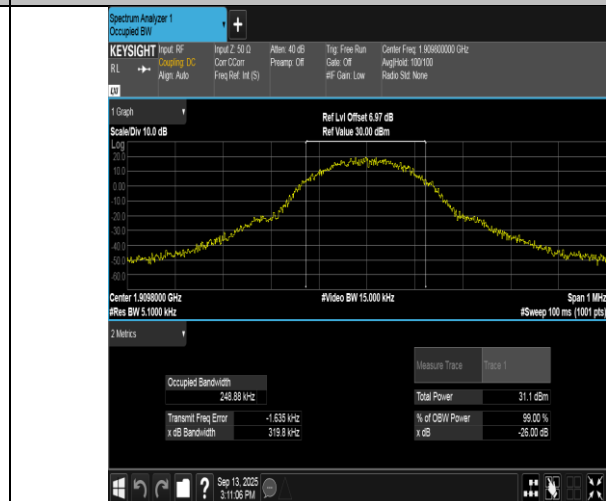
EGPRS1900-810-2-PASS
