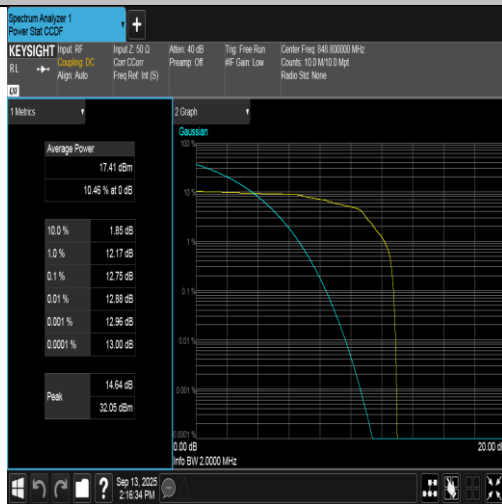
EGPRS850-251-8-PASS
