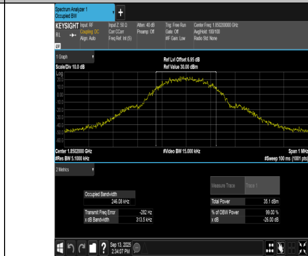
GSM1900-512-0-PASS
