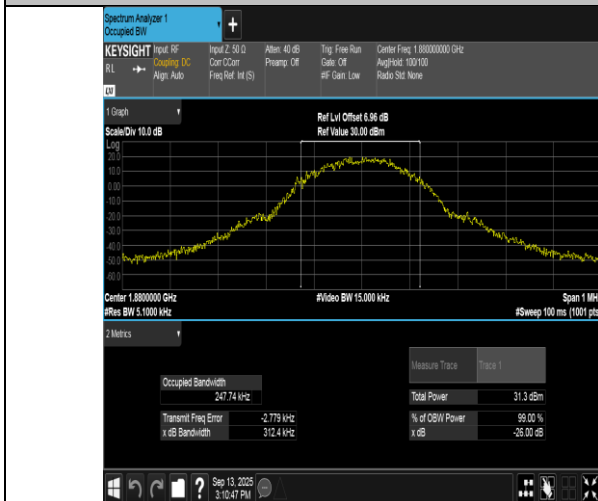
EGPRS1900-661-2-PASS
