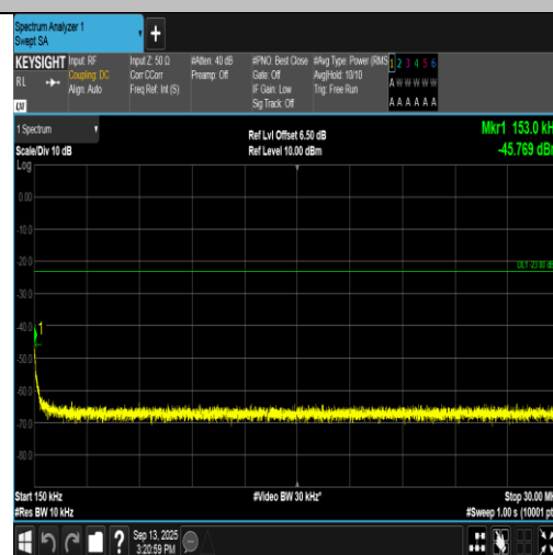
GPRS850-251-5-0.15~30MHz-PASS
