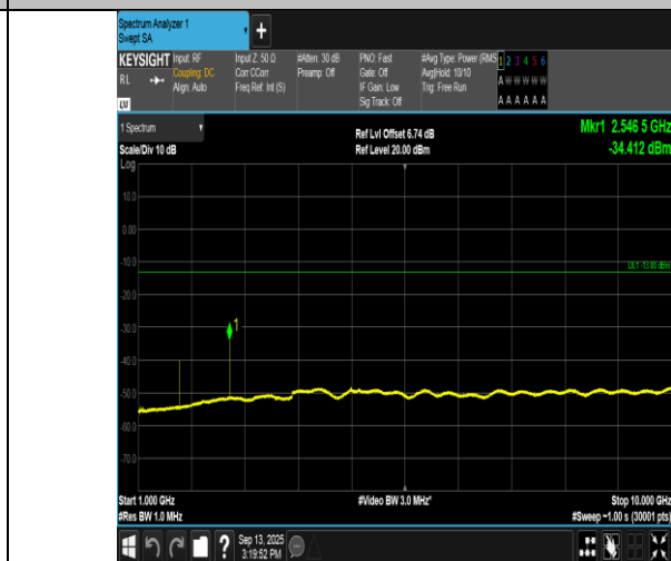
GSM850-251-5-1000~10000MHz-PASS
