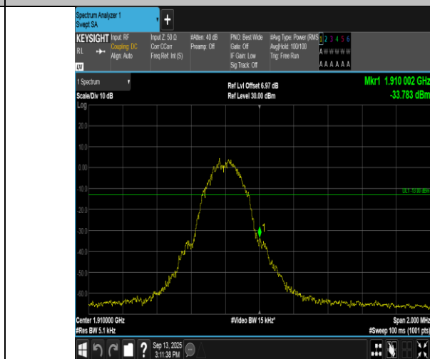
EGPRS1900-810-2-PASS
