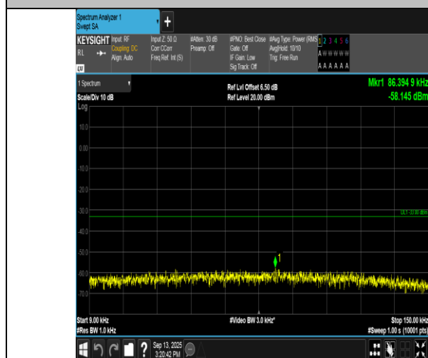
GPRS850-251-5-0.009~0.15MHz-PASS
