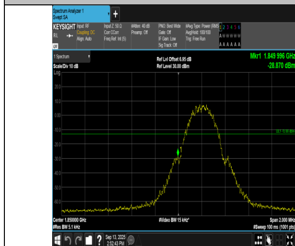
GPRS1900-512-0-PASS
