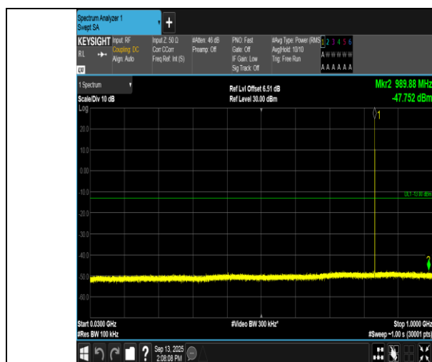
GPRS850-190-5-30~1000MHz-PASS
