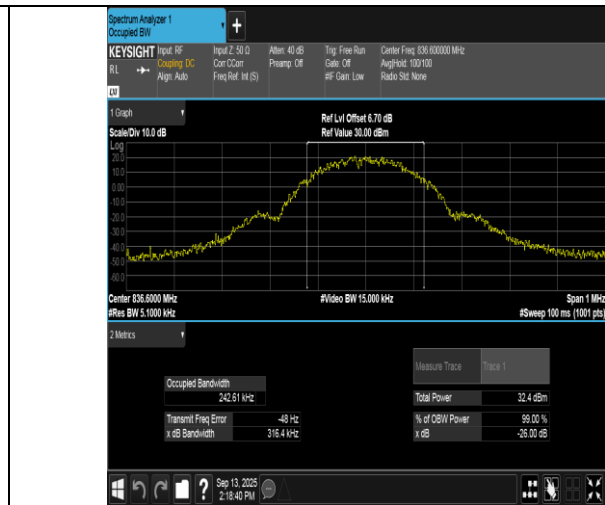
EGPRS850-190-8-PASS
