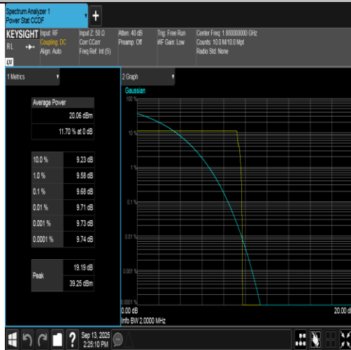
GSM1900-661-0-PASS
