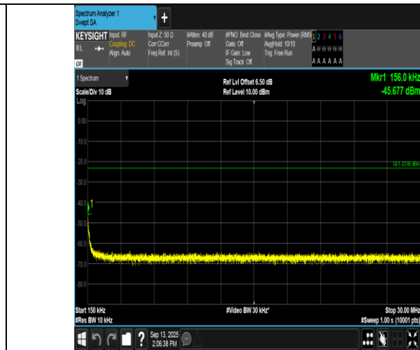
GPRS850-128-5-0.15~30MHz-PASS
