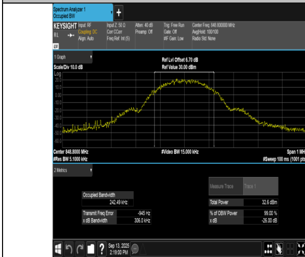
EGPRS850-251-8-PASS
