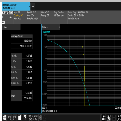
GPRS1900-810-0-PASS
