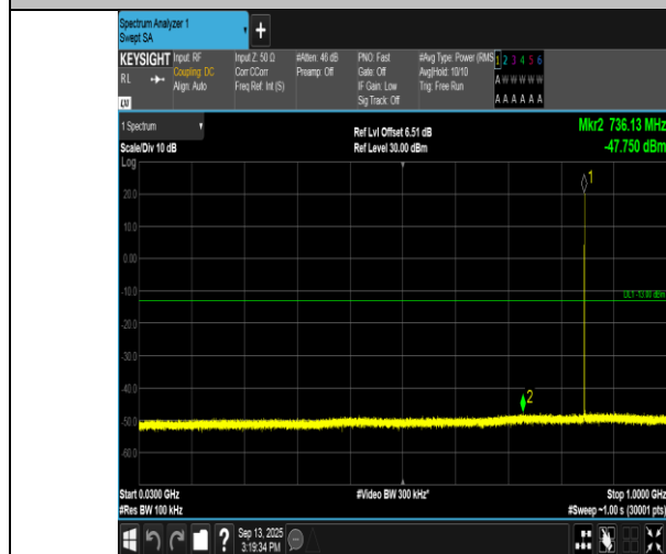
GSM850-251-5-30~1000MHz-PASS
