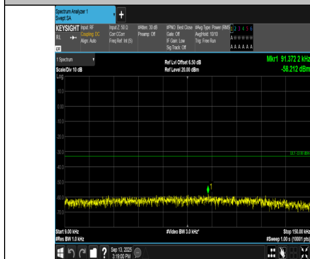
GSM850-251-5-0.009~0.15MHz-PASS
