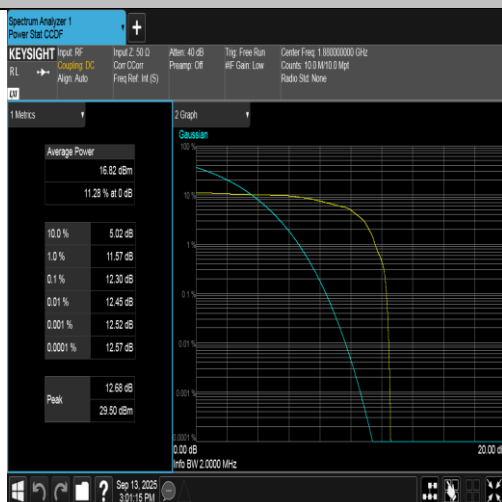
EGPRS1900-661-2-PASS
