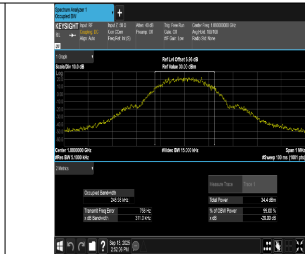
GPRS1900-661-0-PASS
