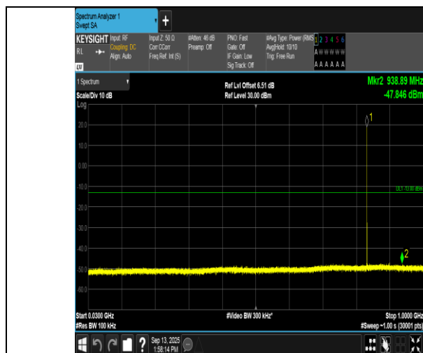
GSM850-190-5-30~1000MHz-PASS
