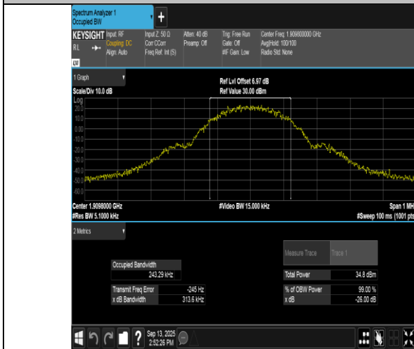
GPRS1900-810-0-PASS
