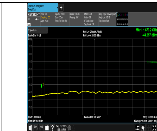
GSM850-190-5-1000~10000MHz-PASS
