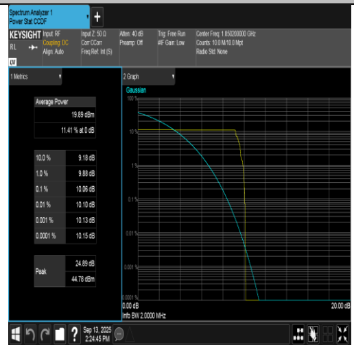
GSM1900-512-0-PASS
