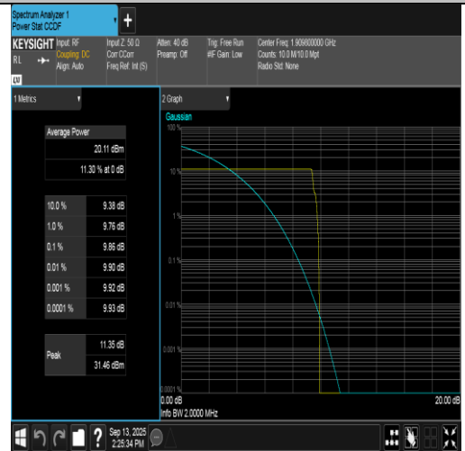
GSM1900-810-0-PASS
