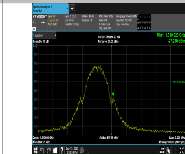
GPRS1900-810-0-PASS
