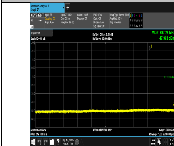
GPRS850-128-5-30~1000MHz-PASS
