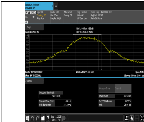
GPRS1900-512-0-PASS
