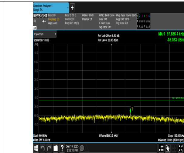
GPRS1900-810-0-0.009~0.15MHz-PASS
