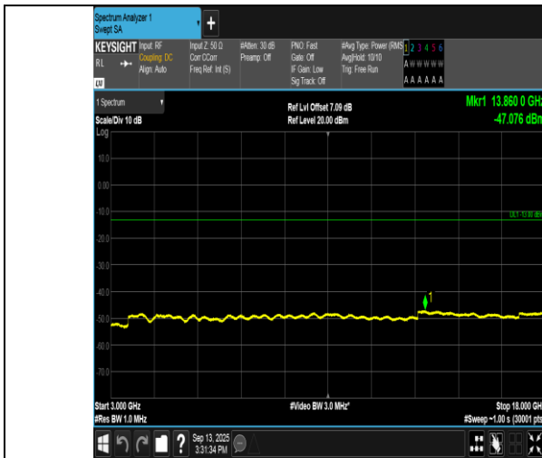
GPRS1900-661-0-3000~18000MHz-PASS
