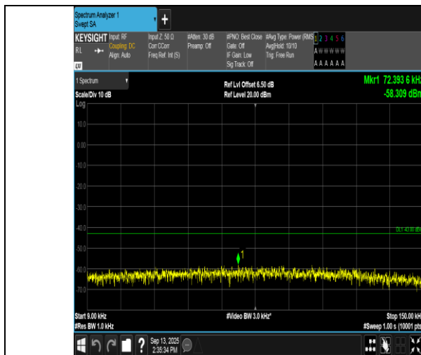
GSM1900-512-0-0.009~0.15MHz-PASS
