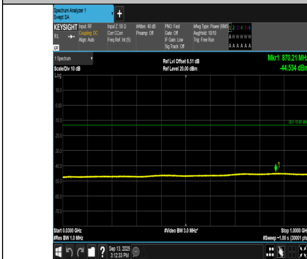
EGPRS1900-512-2-30~1000MHz-PASS
