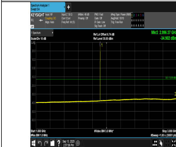
GPRS1900-810-0-1000~3000MHz-PASS
