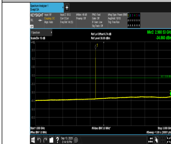
EGPRS1900-661-2-1000~3000MHz-PASS
