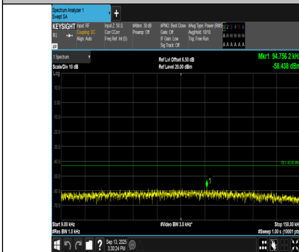
GPRS1900-661-0-0.009~0.15MHz-PASS
