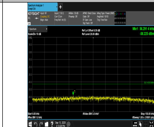
EGPRS1900-661-2-0.009~0.15MHz-PASS
