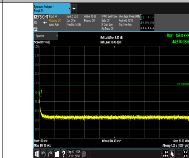
EGPRS1900-810-2-0.15~30MHz-PASS
