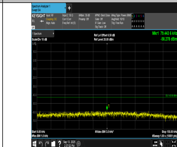
GSM1900-661-0-0.009~0.15MHz-PASS
