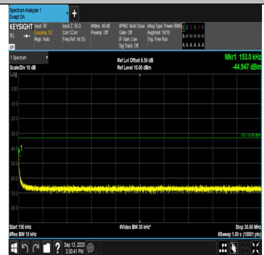
GPRS1900-661-0-0.15~30MHz-PASS
