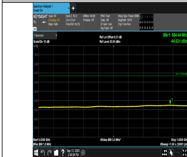
GSM1900-512-0-30~1000MHz-PASS
