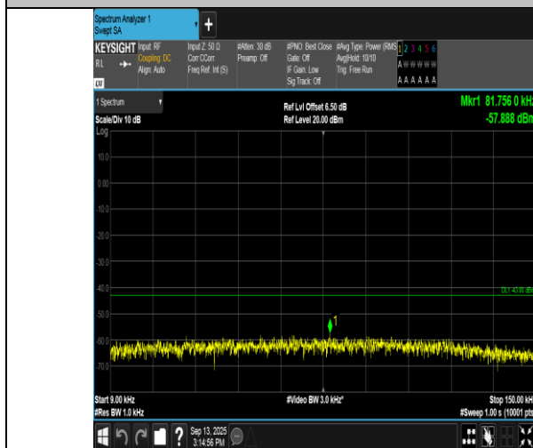
EGPRS1900-810-2-0.009~0.15MHz-PASS
