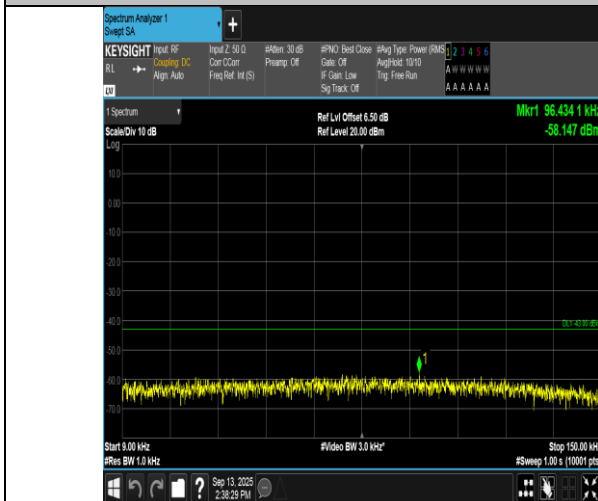
GSM1900-810-0-0.009~0.15MHz-PASS
