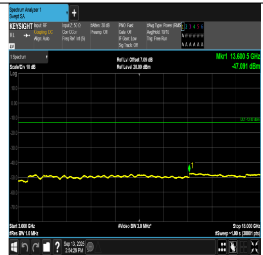
GPRS1900-512-0-3000~18000MHz-PASS
