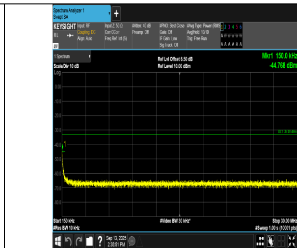
GSM1900-512-0-0.15~30MHz-PASS
