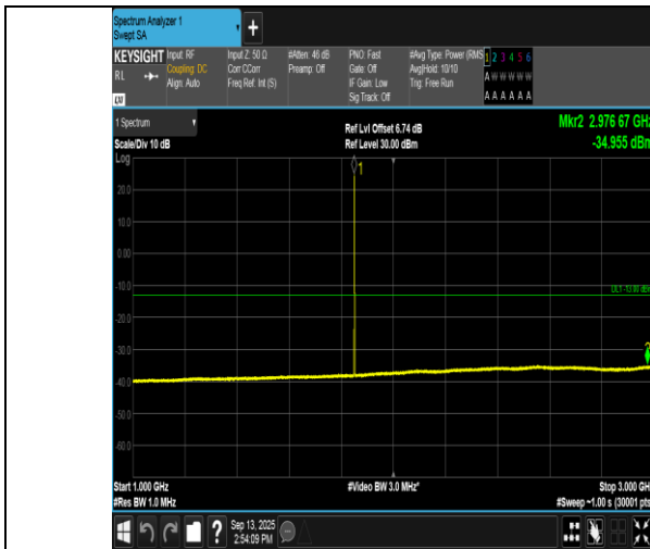
GPRS1900-512-0-1000~3000MHz-PASS
