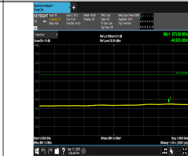
GPRS1900-810-0-30~1000MHz-PASS
