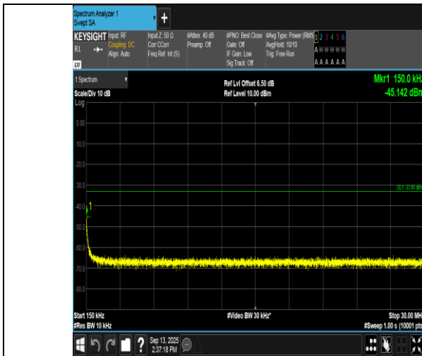
GSM1900-661-0-0.15~30MHz-PASS
