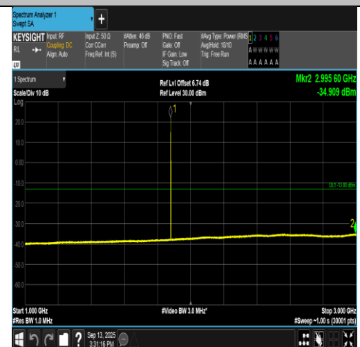
GPRS1900-661-0-1000~3000MHz-PASS
