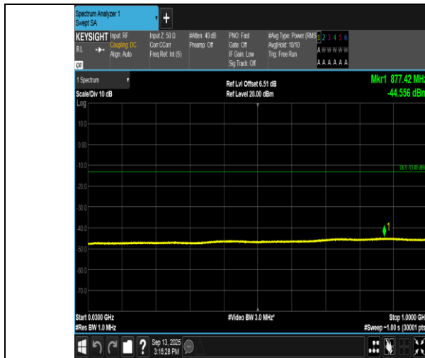
EGPRS1900-810-2-30~1000MHz-PASS
