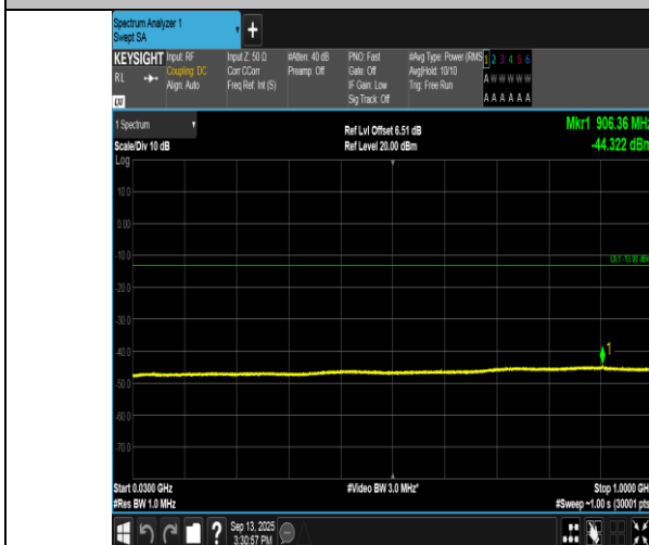
GPRS1900-661-0-30~1000MHz-PASS
