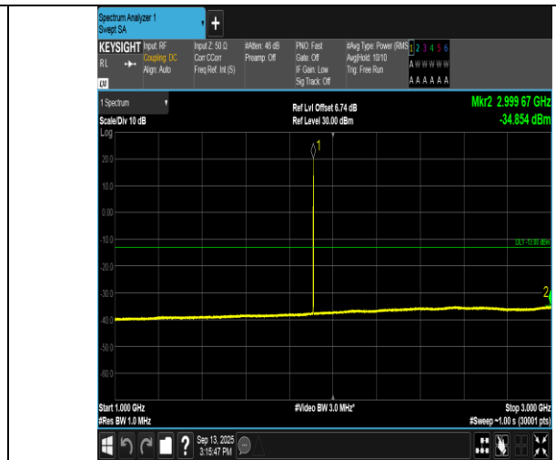
EGPRS1900-810-2-1000~3000MHz-PASS
