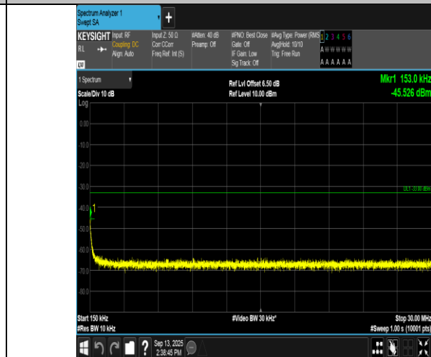
GSM1900-810-0-0.15~30MHz-PASS
