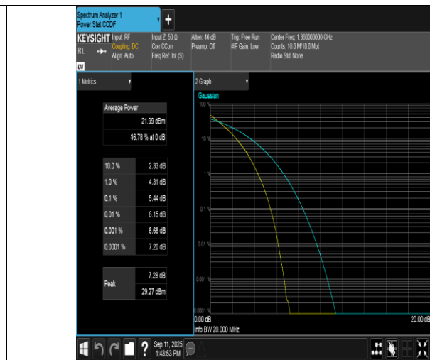
Band2-20MHz-QPSK-18700-100RB#0-PASS
