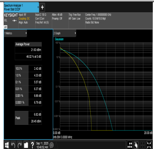
Band2-3MHz-QPSK-18900-15RB#0-PASS
