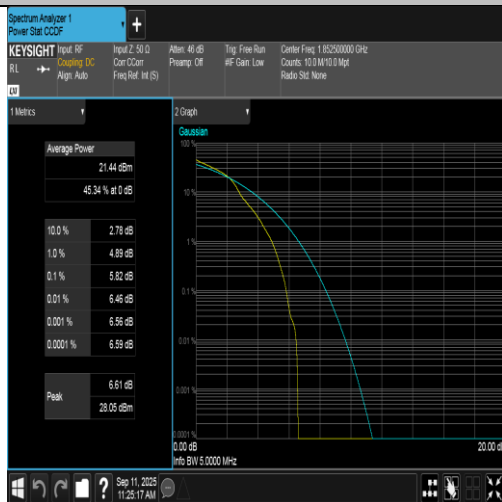
Band2-5MHz-16QAM-18625-1RB#0-PASS
