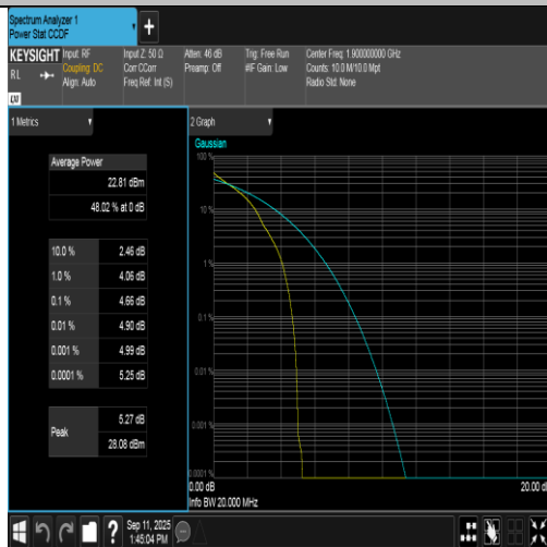
Band2-20MHz-QPSK-19100-1RB#0-PASS
