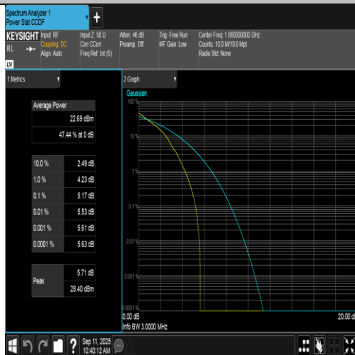
Band2-3MHz-QPSK-18900-1RB#0-PASS
