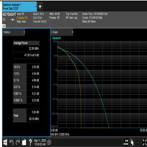
Band2-3MHz-QPSK-18615-1RB#0-PASS
