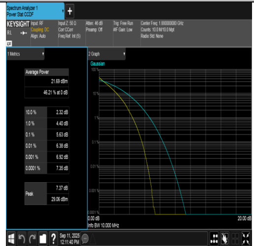
Band2-10MHz-QPSK-18900-50RB#0-PASS
