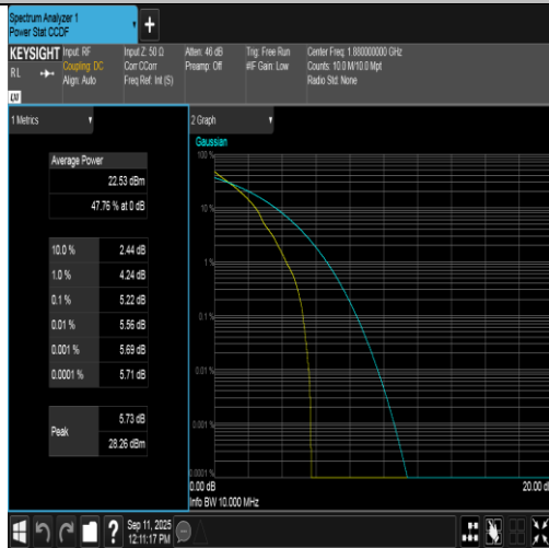
Band2-10MHz-QPSK-18900-1RB#0-PASS
