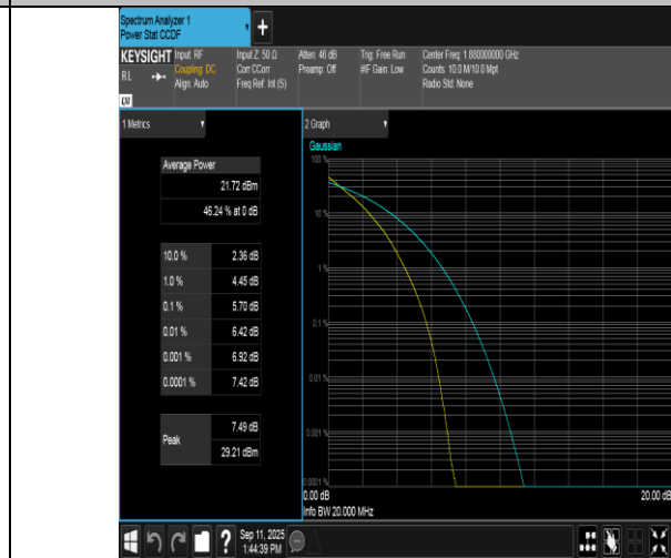
Band2-20MHz-QPSK-18900-100RB#0-PASS
