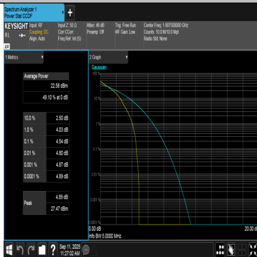
Band2-5MHz-QPSK-19175-1RB#0-PASS
