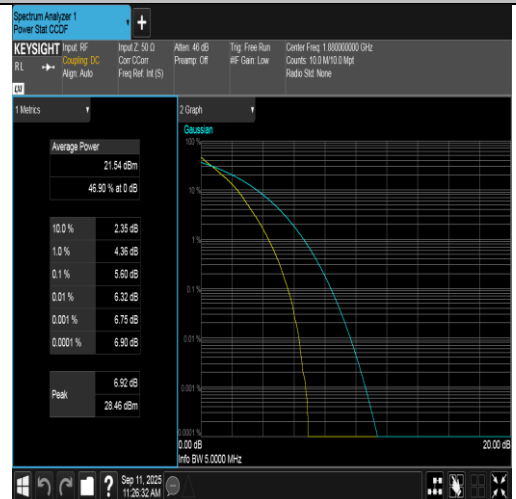
Band2-5MHz-QPSK-18900-25RB#0-PASS
