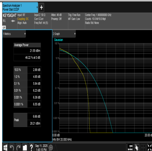
Band2-20MHz-16QAM-19100-1RB#0-PASS
