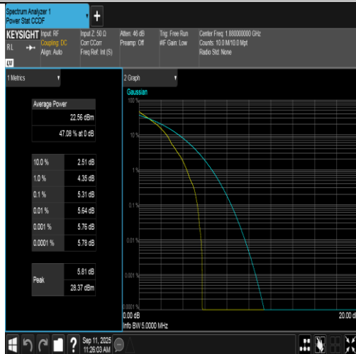
Band2-5MHz-QPSK-18900-1RB#0-PASS
