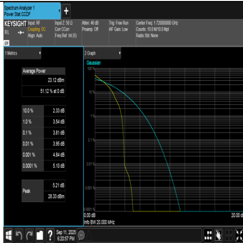
Band4-20MHz-QPSK-20050-1RB#0-PASS
