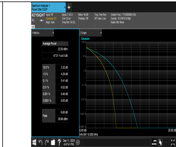
Band4-10MHz-QPSK-20000-50RB#0-PASS
